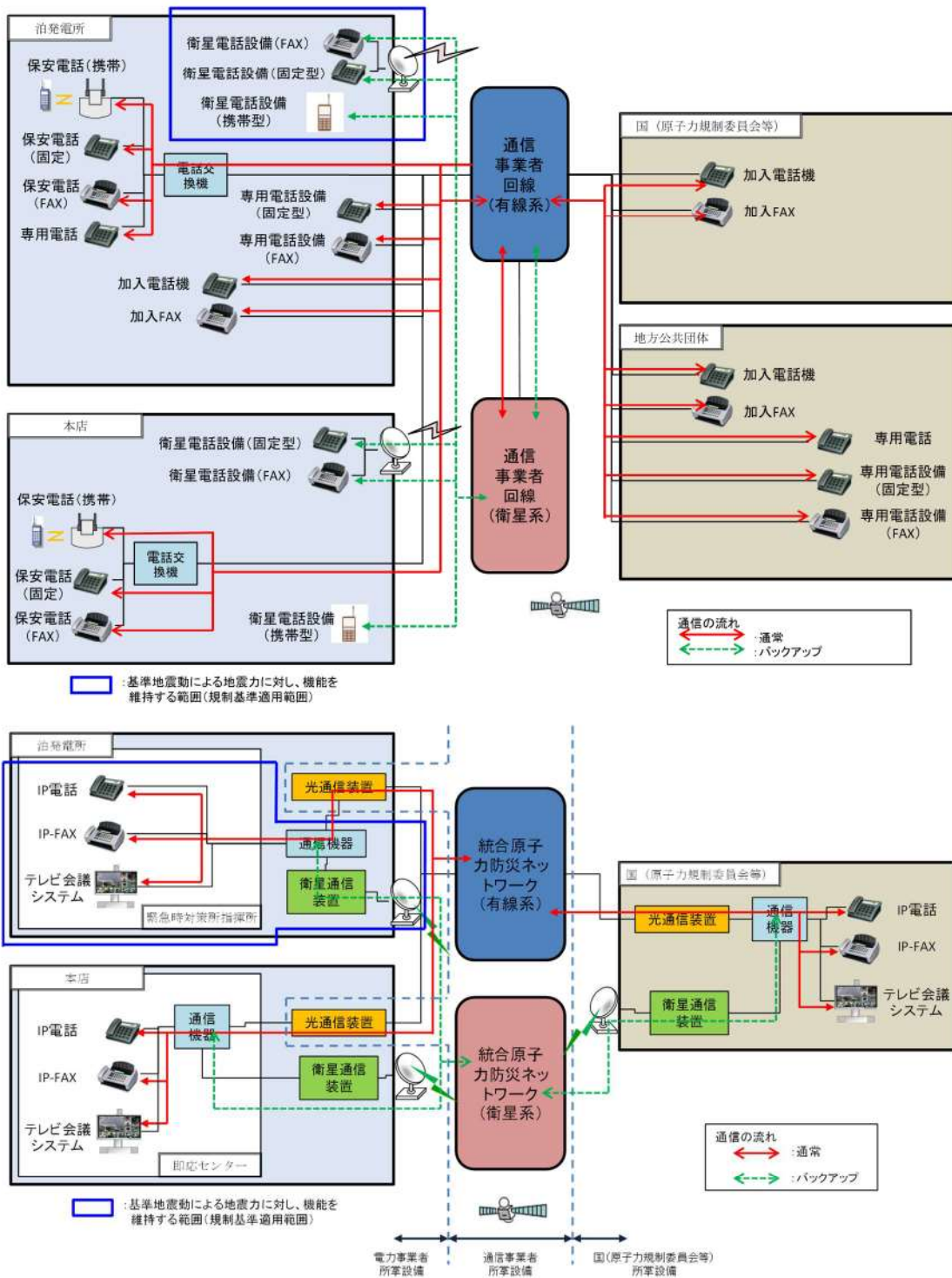
図 4-8 通信連絡設備の耐震設計範囲
