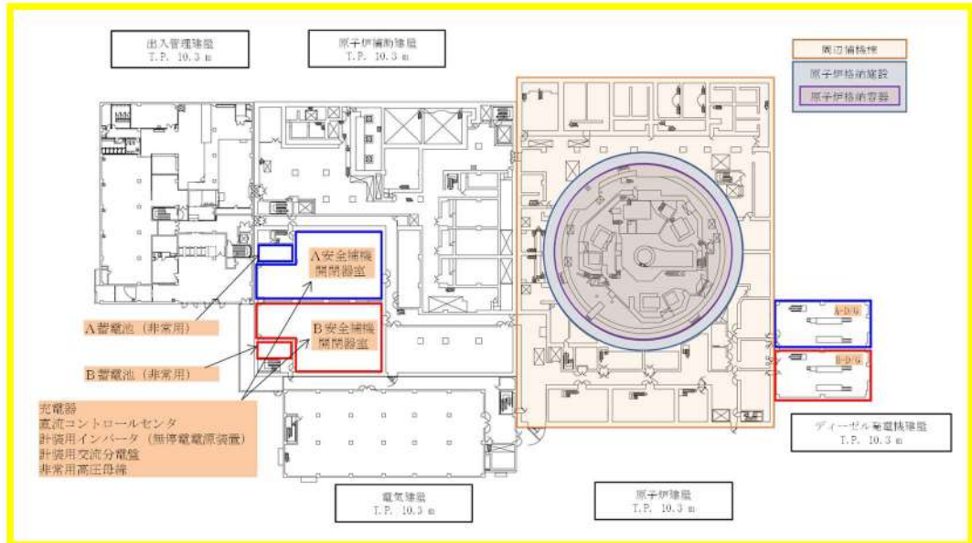
第 2.3.1.1 図 非常用電源設備の配置
