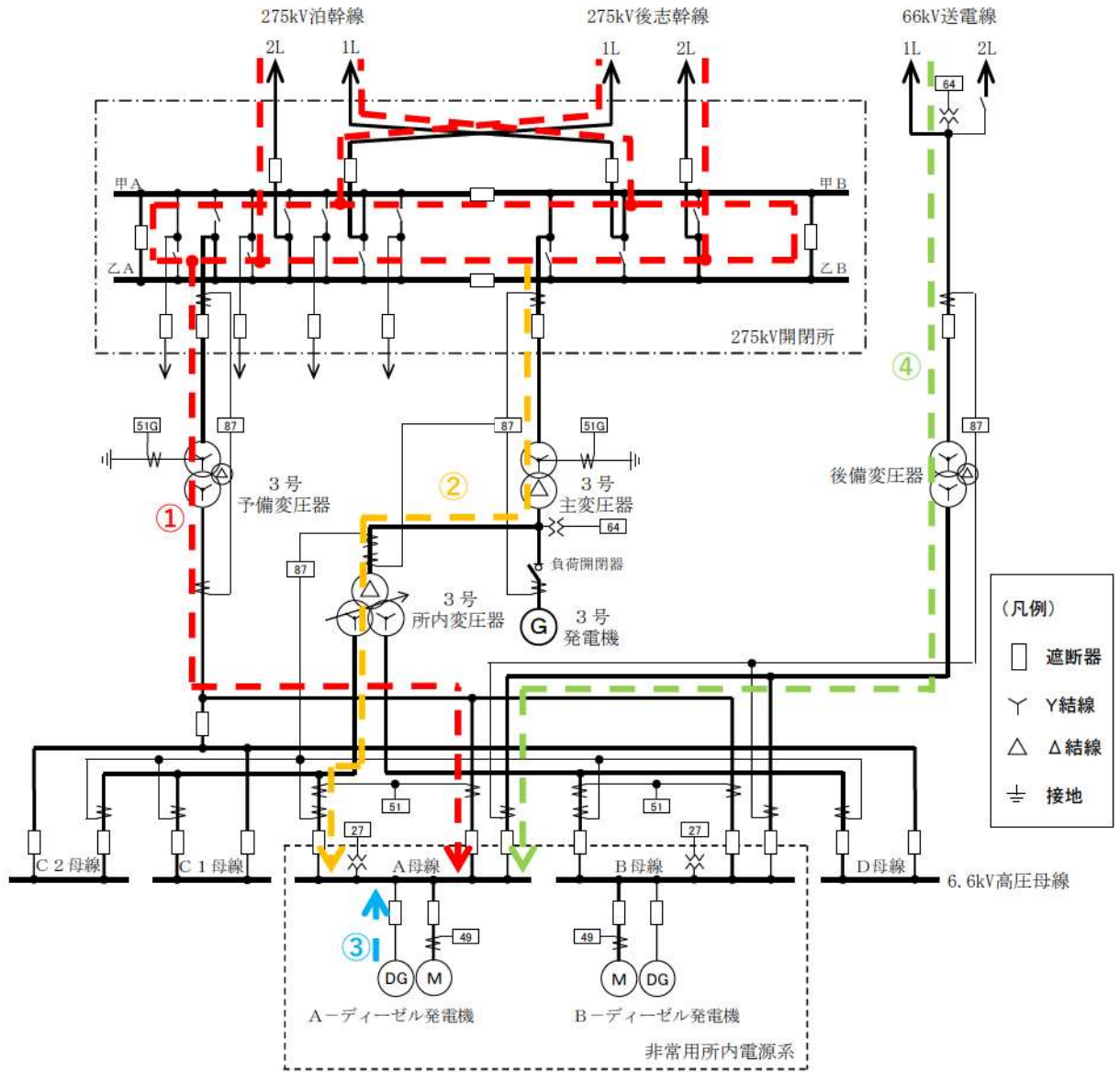
第 2. 2. 1. 9 図 非常用高圧母線への電力供給
