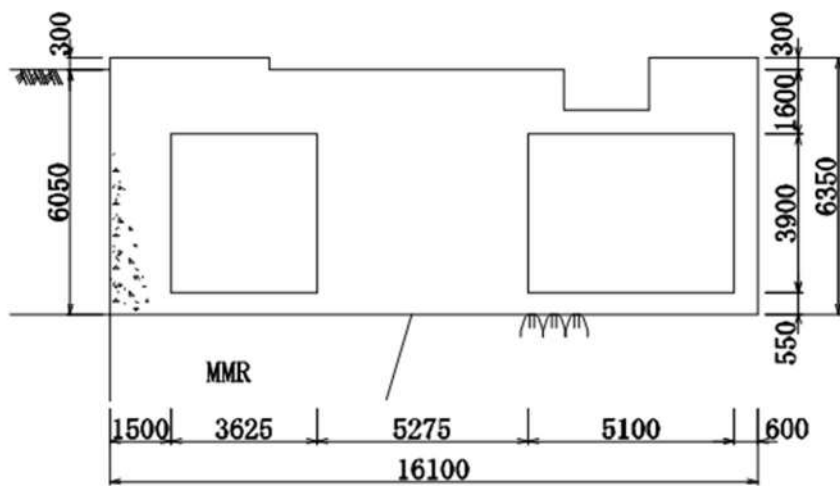
A-A 断面图
