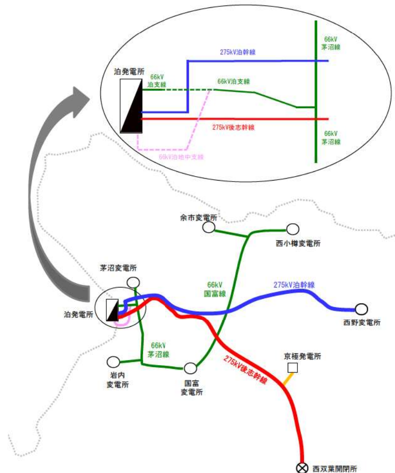
第 2.2.3.1 図 送電線ルート
