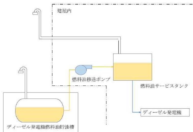
第 1-26 図：油タンクのベント管設置の概要
