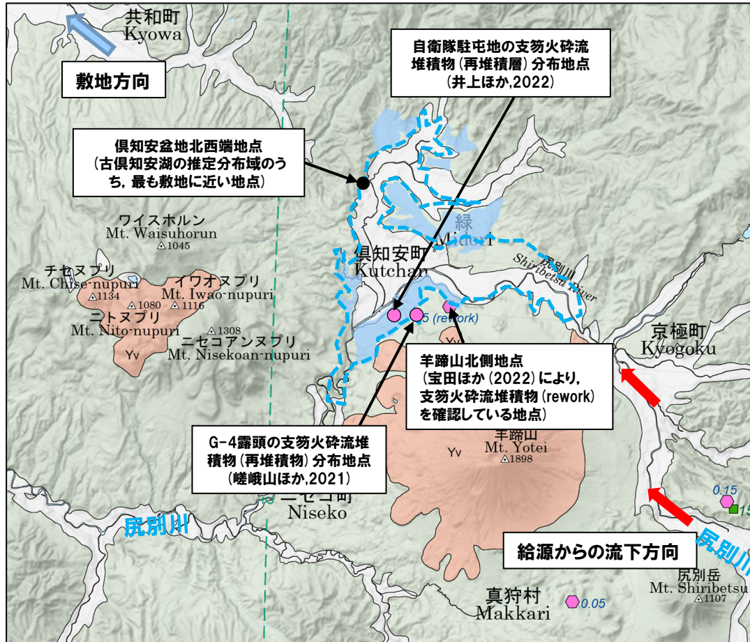
羊蹄山周辺の支笏火砕流堆積物の分布 (宝田ほか (2022) に加筆)
