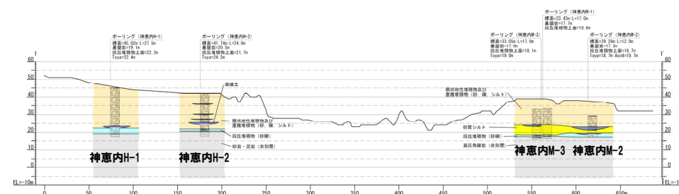
1-1' 断面
