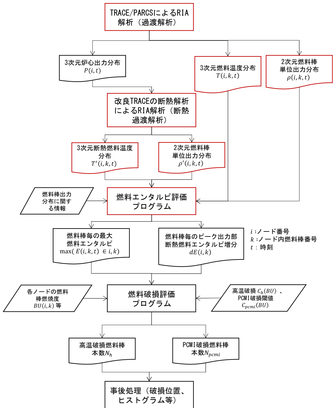
図1 TRACE/PARCS コードを用いた燃料棒破損評価の流れ (朱枠: 改良範囲)
