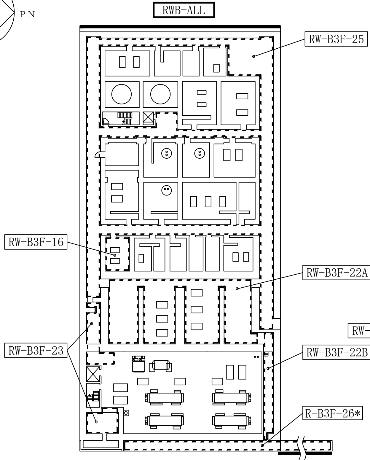
廃棄物処理建屋 T.M.S.L. - 6100
