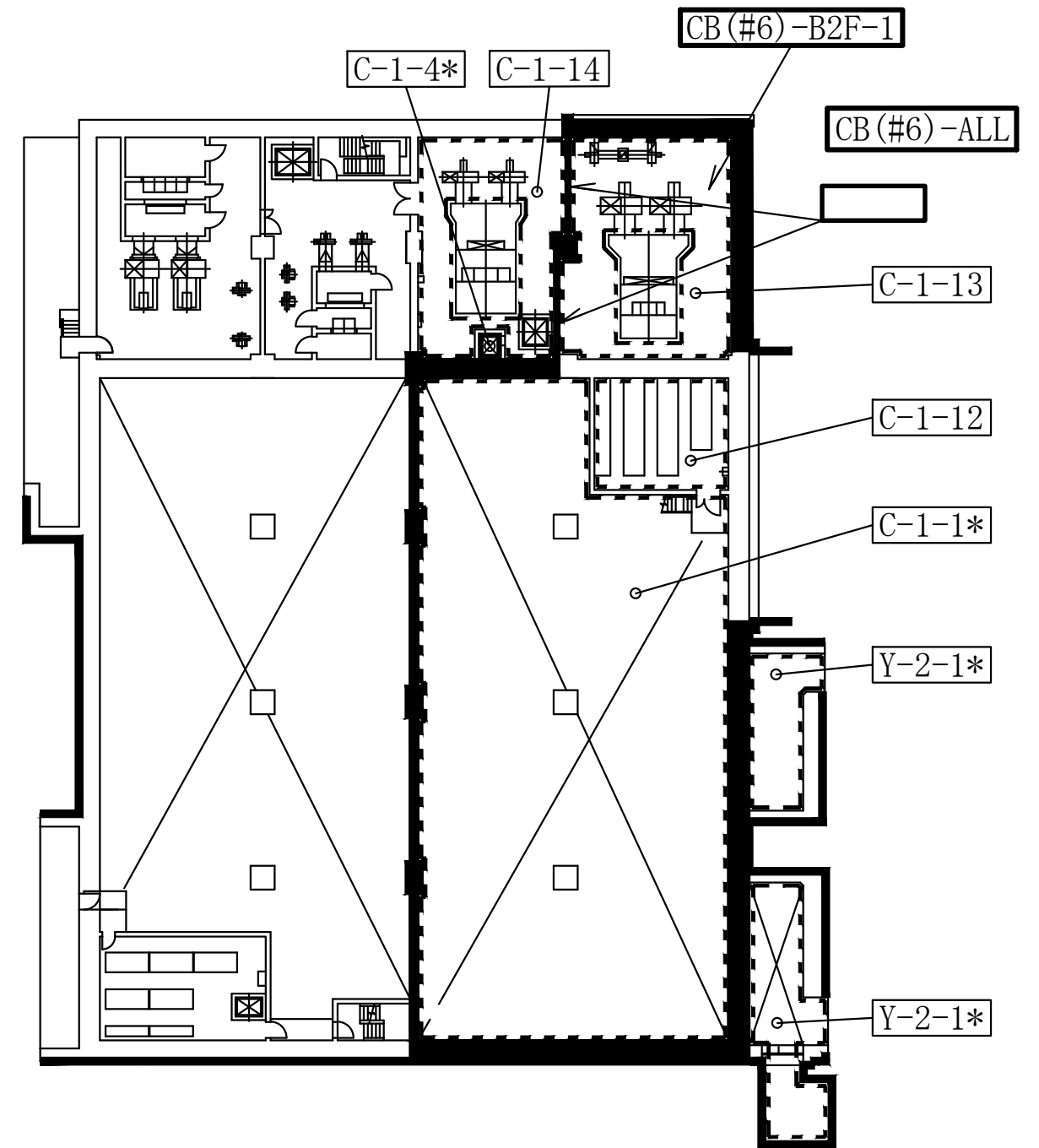
コントロール建屋 T.M.S.L. 1000
