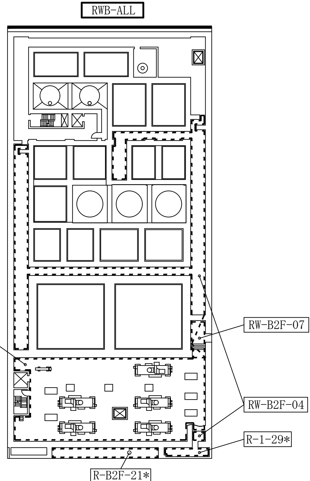
廃棄物処理建屋 T.M.S.L. - 1100
