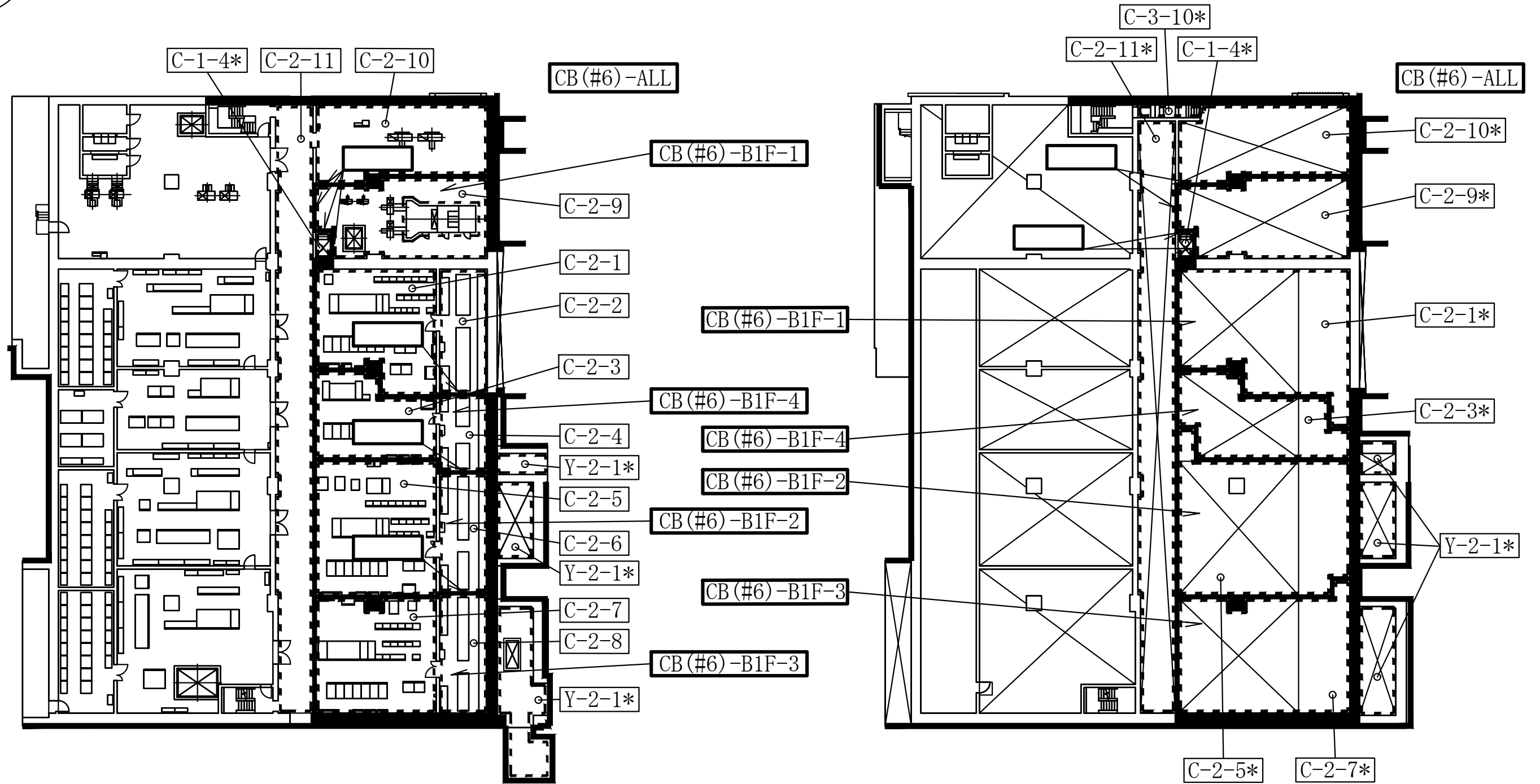
コントロール建屋 T.M.S.L. 6500
