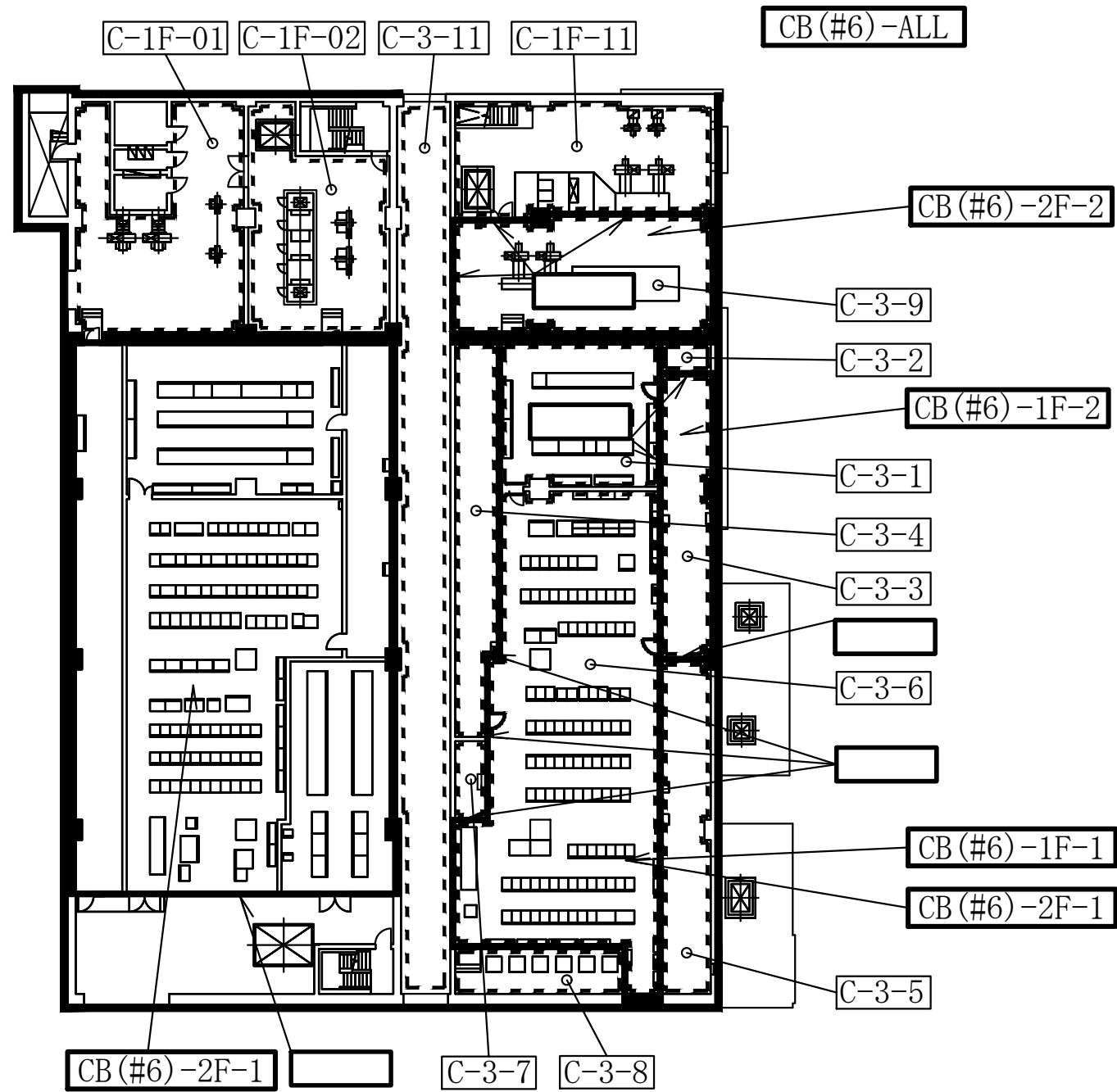
コントロール建屋 T.M.S.L. 12300
