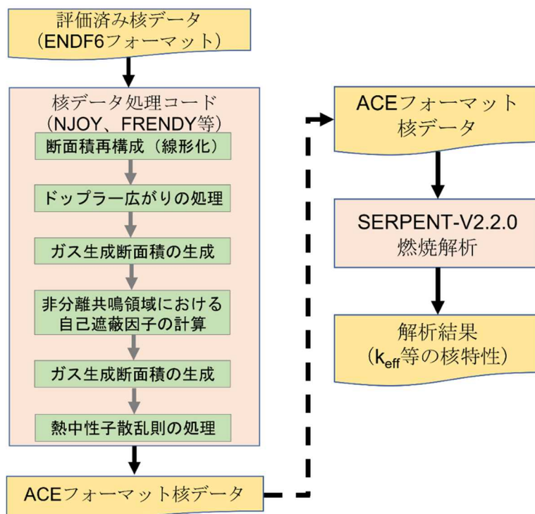
図1 核データ処理コードによる処理及びSERPENTコードによる燃焼解析の流れ
