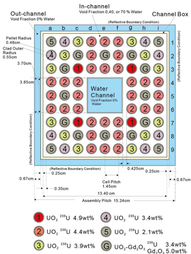
図2 Phase III-C ベンチマークにおける BWR 9×9 燃料集合体モデル
