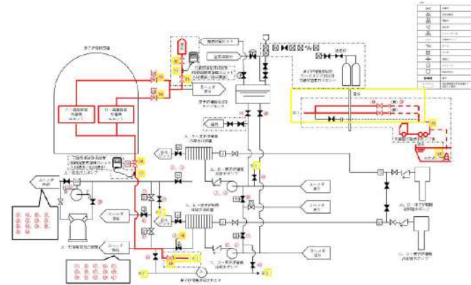
図 50-4-3 可搬型大型送水ポンプ車を用いたC、D-格納容器再循環ユニットによる格納容器内自然対流冷却（建屋外接続口を使用する場合）
