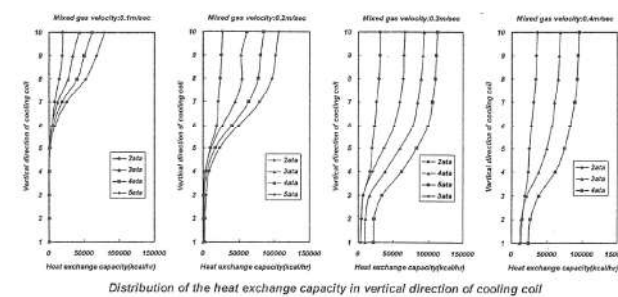
図4. 3-1 冷却コイル高さ方向の除熱分布
