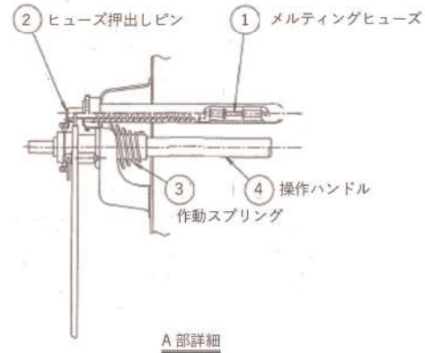
図1-5 ダクト開放機構概略図
