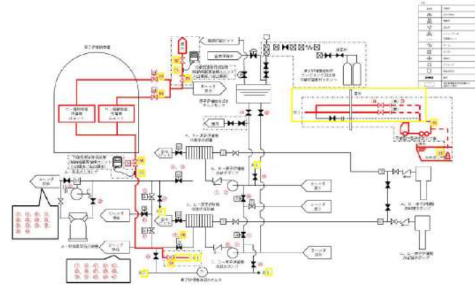
図49-4-3 格納容器内自然対流冷却（建屋外接端口を使用する場合）
