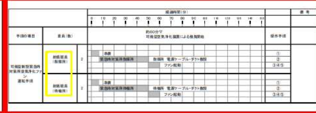
図3.2-12 可搬型新設緊急時対策所空気浄化ファンによる正圧化 (ブルーム通過前) のタイムチャート (操作手順 a.)
