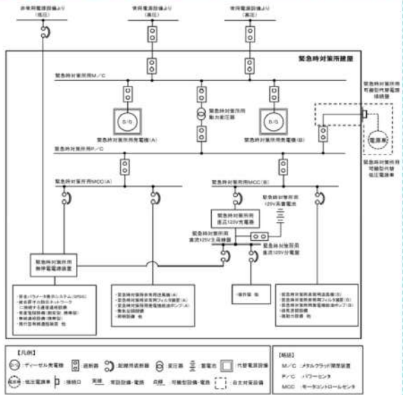
第2.2-1図 緊急時対策所 単線結線図
