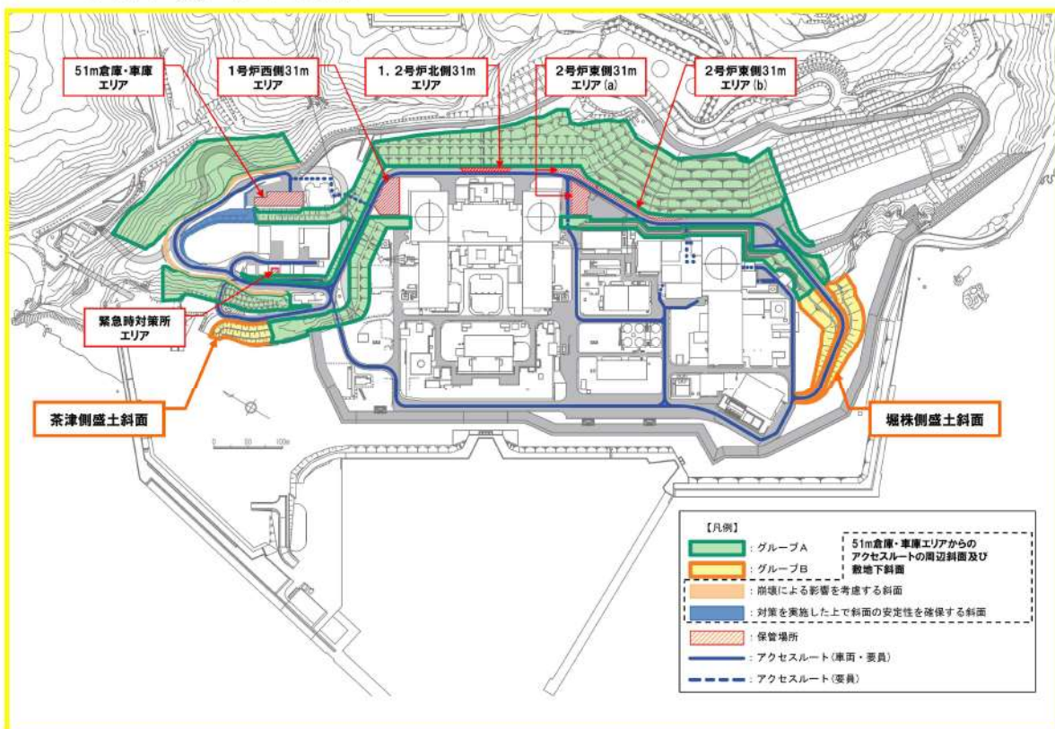
第5.1-1図 保管場所及びアクセスルートに影響を及ぼすおそれのある斜面の分類位置図
