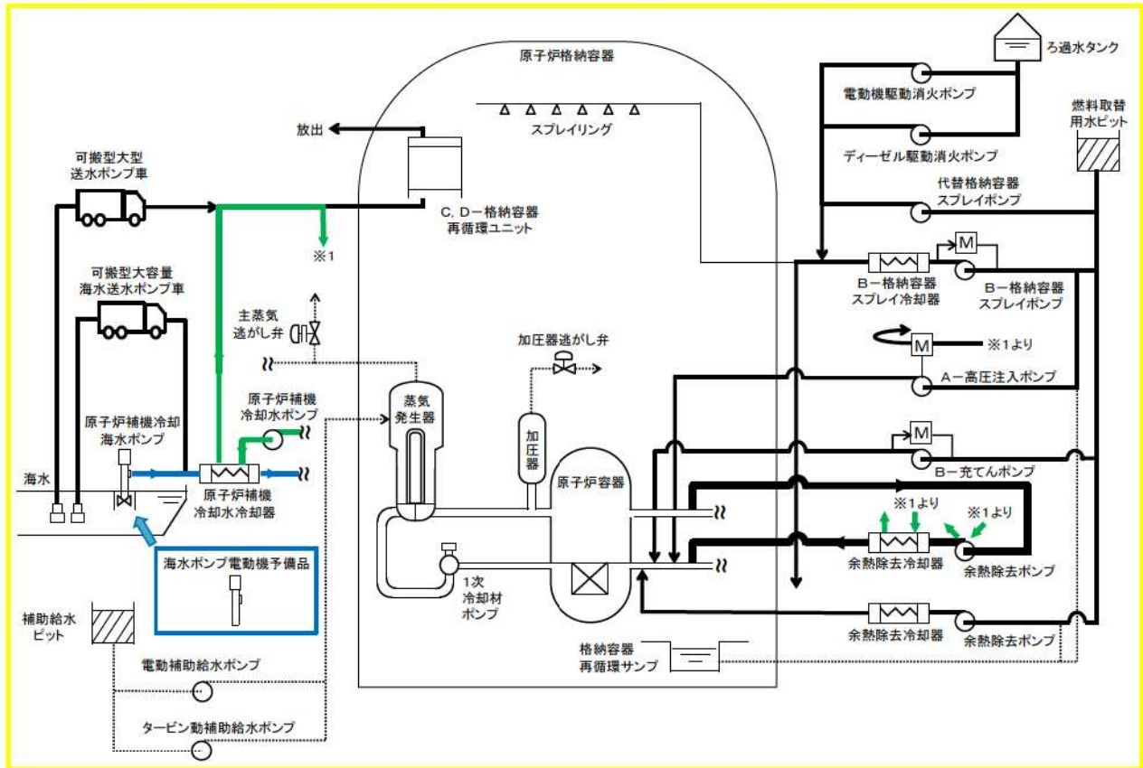
図5 概略系統図
