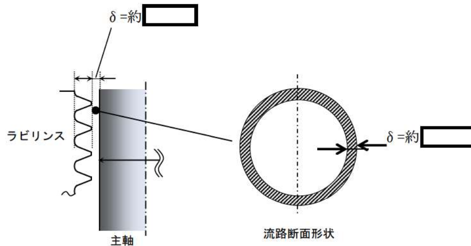
図1 RCPラビリンズ部流路の断面形状
