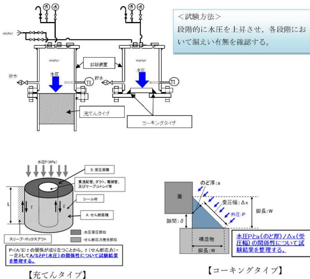
図9 シリコンシーラント及び充てんシール材の耐水圧試験概要図
