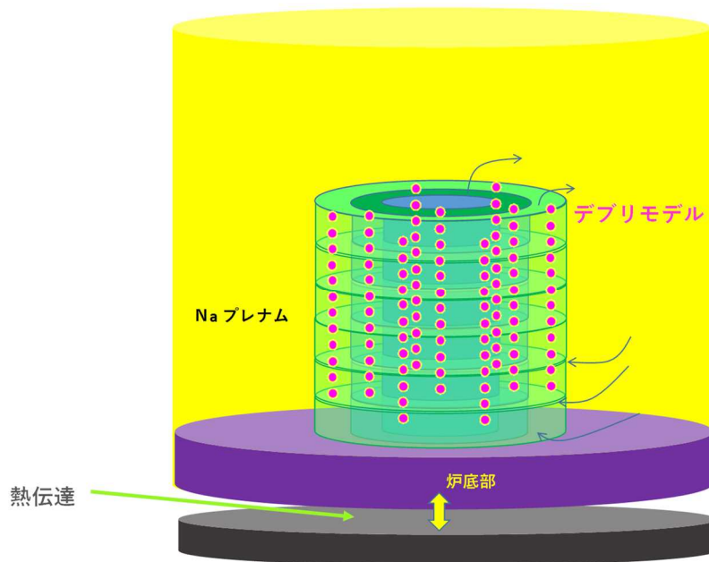
図1 3次元デブリベッド冷却評価モデルの概念（“SPH_D10 試験モデル”）
