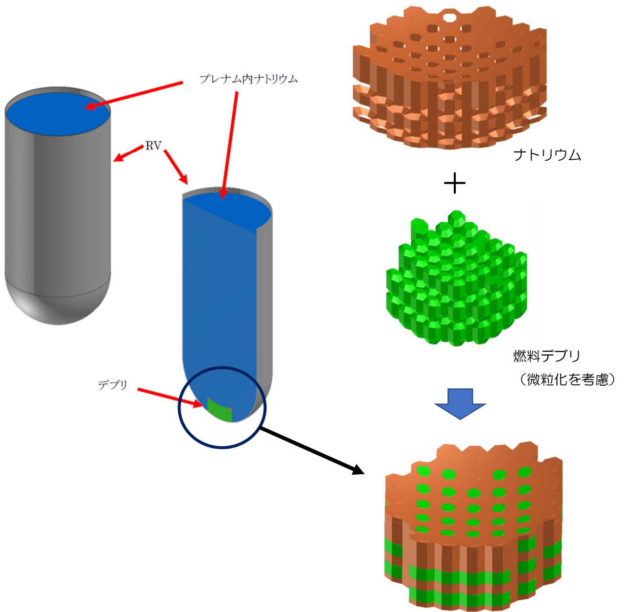
図3 “実機体系モデル”
