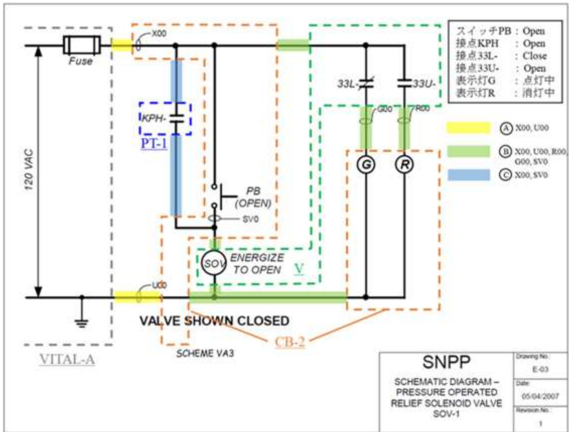
図 4.1-2 展開接続図 (EWD) の色分けのイメージ例 (*)2
