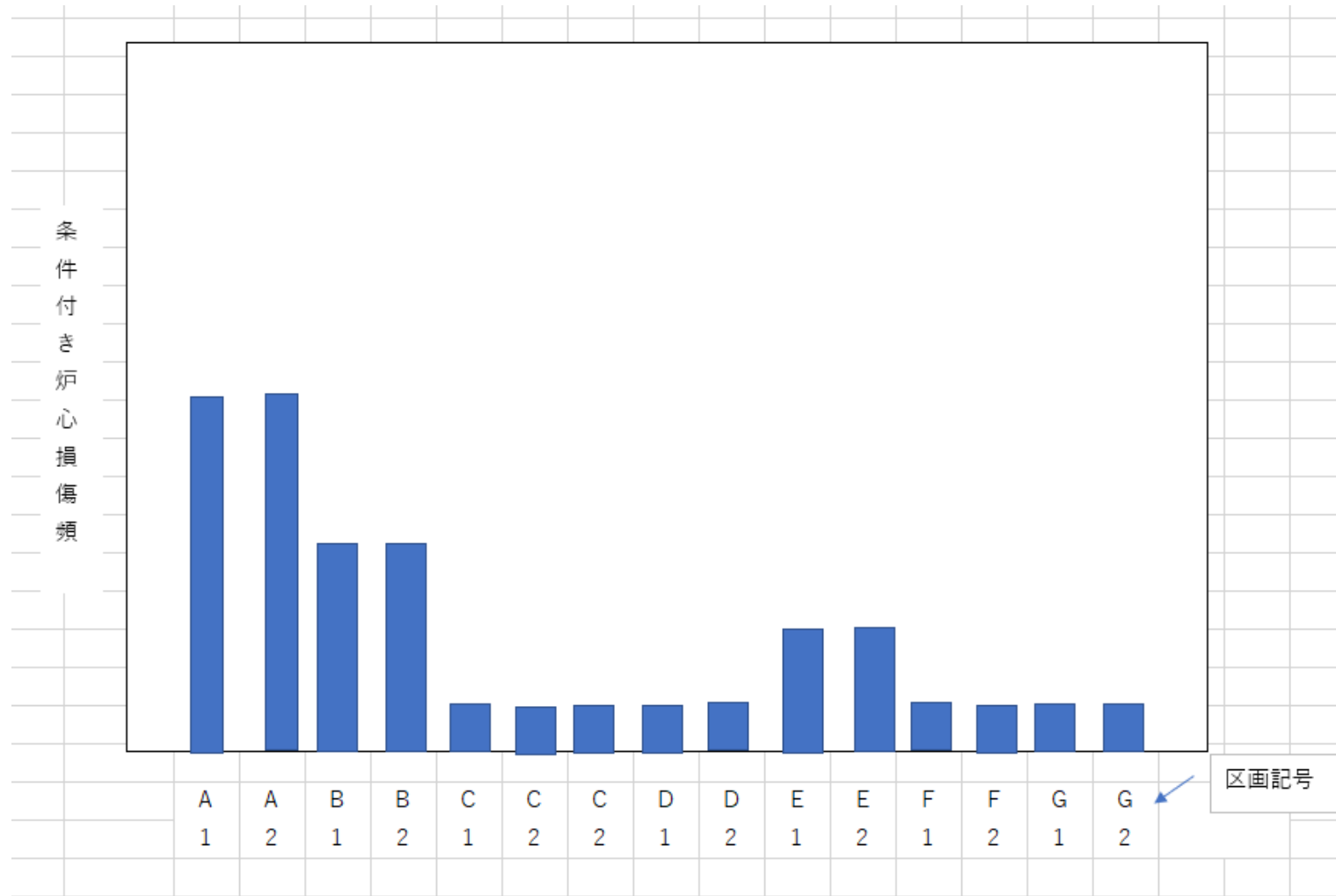
図 4. 4-1 起因事象（手動停止）における各区画での条件付き炉心損傷頻度(例)
