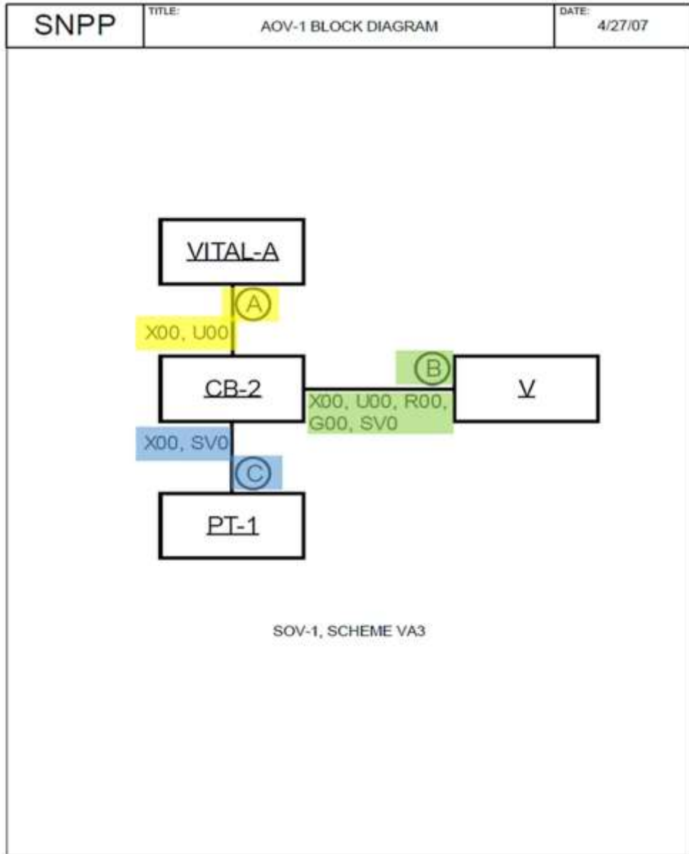
図 4.1-1 配線接続図 (EBD) の色分けのイメージ例 (*2)
