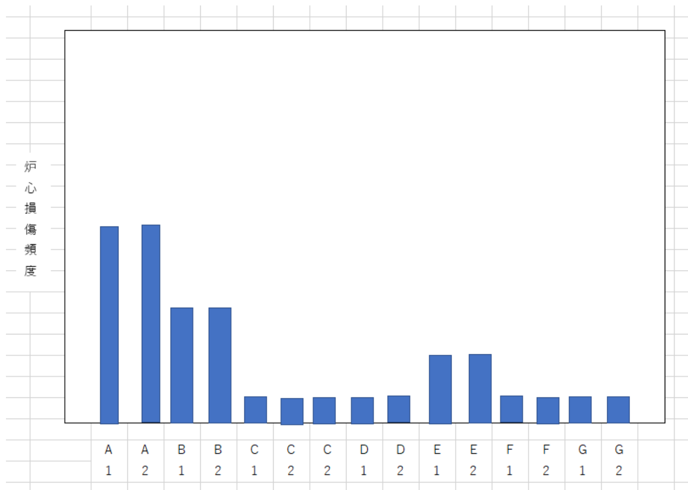
図 4.4-2 起因事象（手動停止）における各区画での炉心損傷頻度(例)
