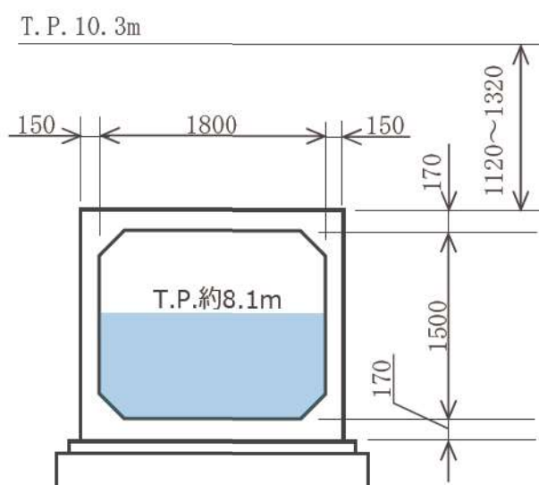
添付 7-6 図 原子炉補機冷却海水放水路 (断面図)
