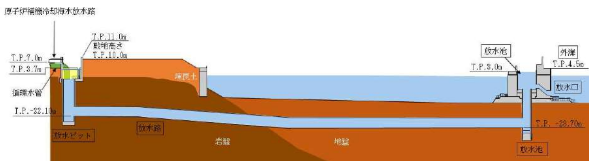
添付 7-8 図 放水路、放水池及び放水口断面図
