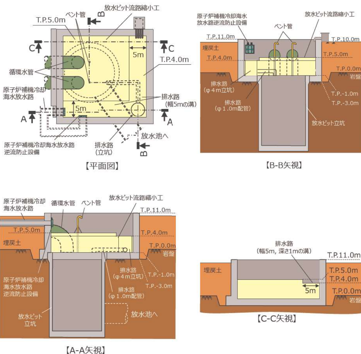
添付 7-7 図 放水ピット（断面図）
