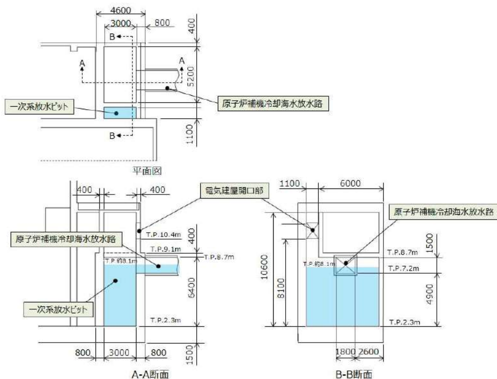
添付7-5図 一次系放水ピット三面図
