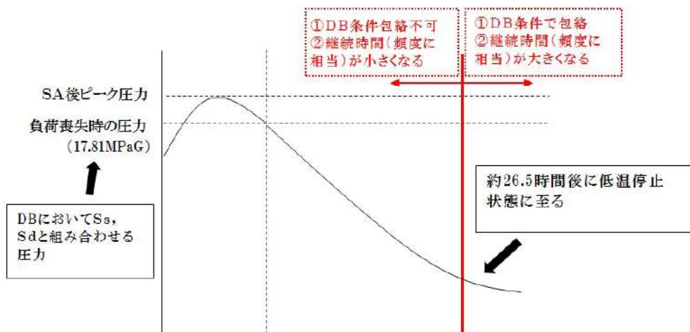
(例：RCPB 圧力推移の概念図)
