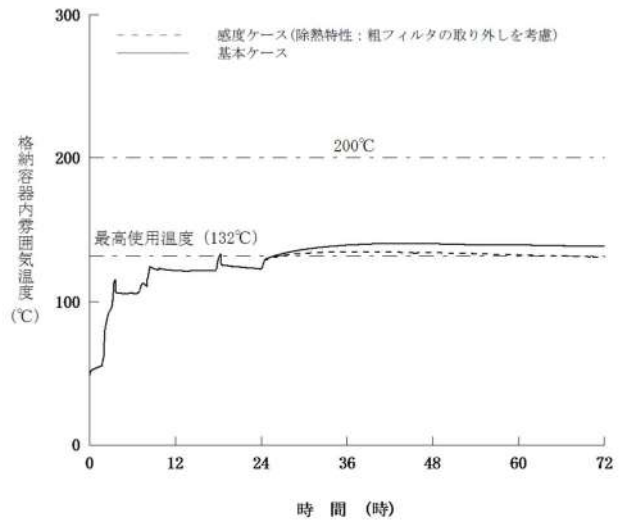
図 12 C/V 過温破損における C/V 温度の時間変化
