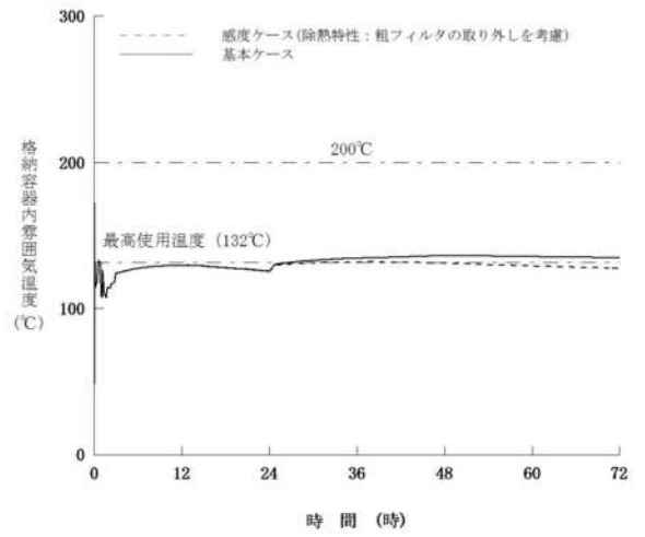
図 10 C/V 過圧破損における C/V 温度の時間変化
