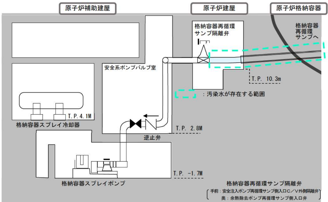
格納容器再循環サンブから格納容器スプレイポンプ、余熱除去ポンプまでのルート図
