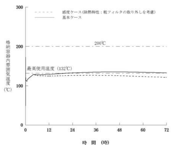
図4 C/V 先行破損における C/V 温度の時間変化
