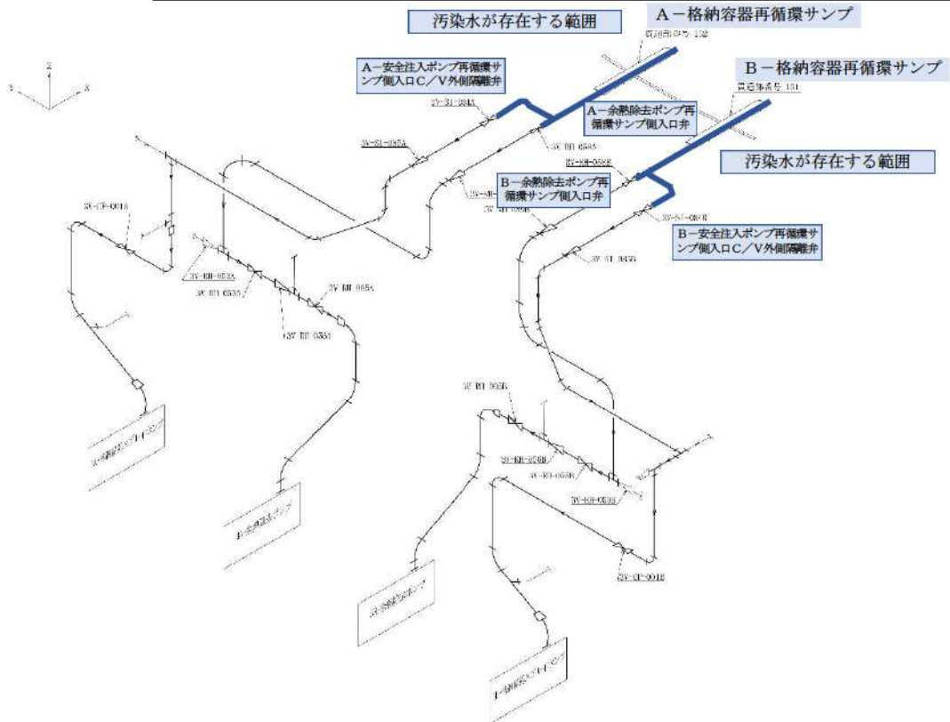
格納容器再循環サンブから格納容器スプレイポンプ、余熱除去ポンプまでのルート図
