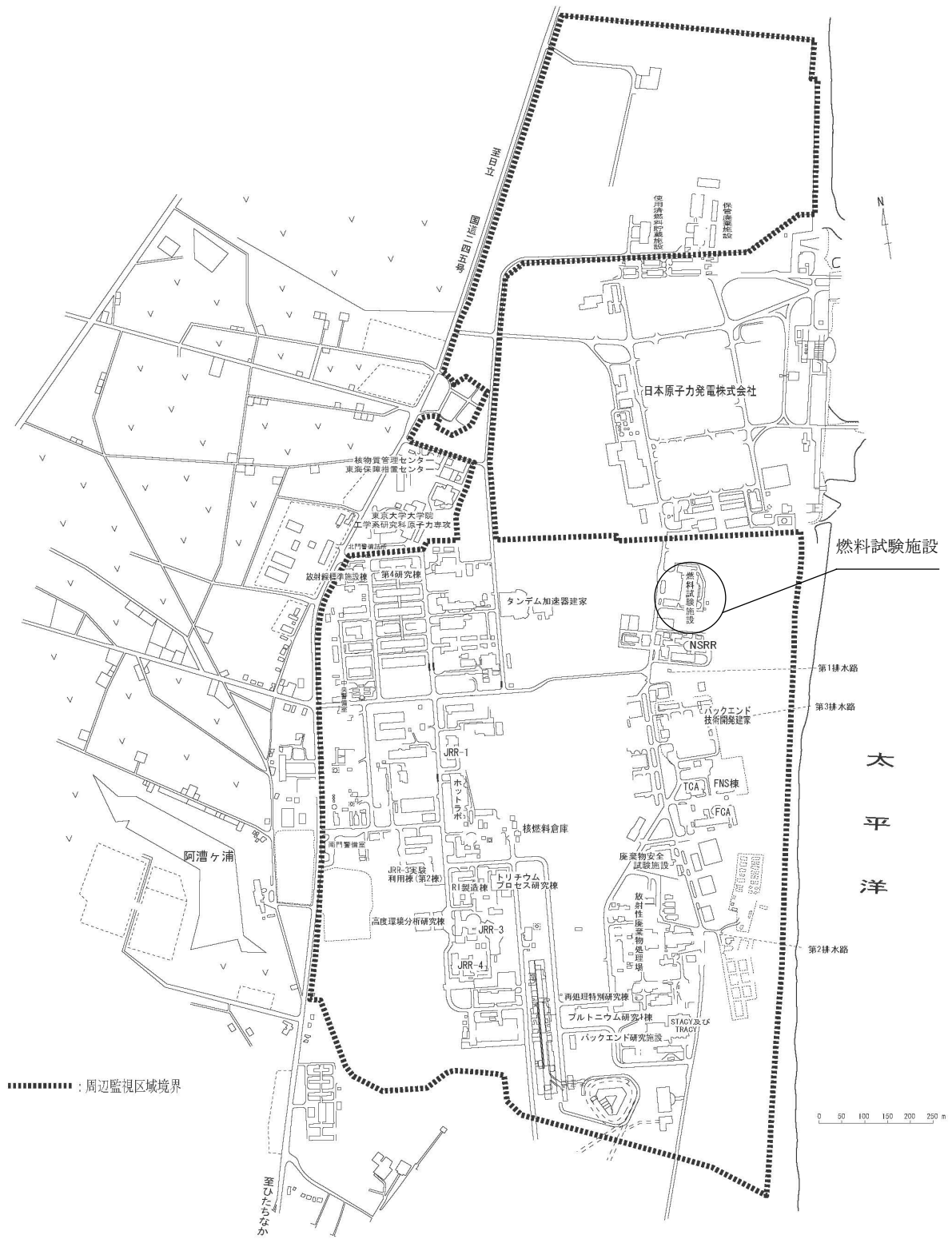
図1 国立研究開発法人日本原子力研究開発機構原子力科学研究所配置図
