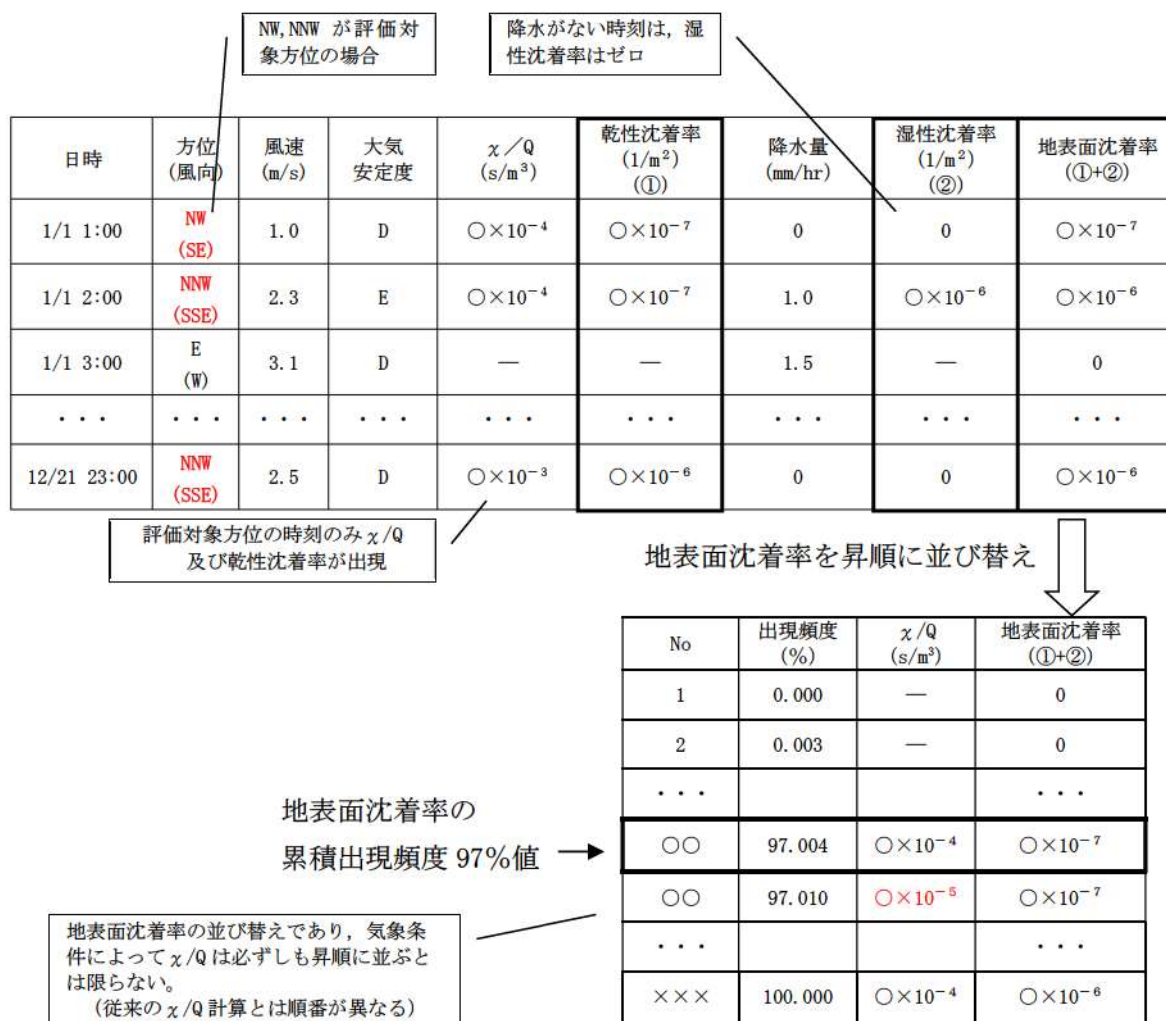
第2図 地表面沈着率の累積出現頻度 97%値の求め方
