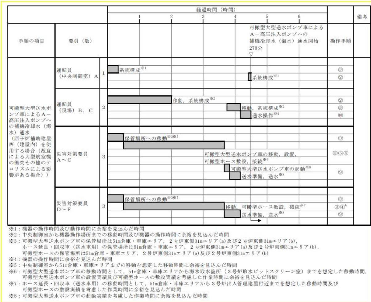
第 1.5.8 図 可搬型大型送水ポンプ車によるA-高圧注入ポンプへの補機冷却水 (海水) 通水 タイムチャート (2/2) (原子炉補助建屋西 (建屋内) 接続口を使用する場合 (故意による大型航空機の衝突その他のテロリズムによる影響がある場合))
