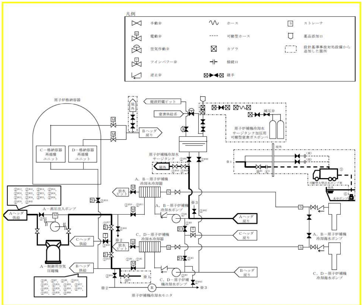
第 1.5.9 図 可搬型大型送水ポンプ車による A-制御用空気圧縮機への補機冷却水（海水）通水 概要図（3/4） （原子炉補助建屋西（建屋内）接続口を使用する場合（故意による大型航空機の衝突その他のテロリズムによる影響がある場合））
