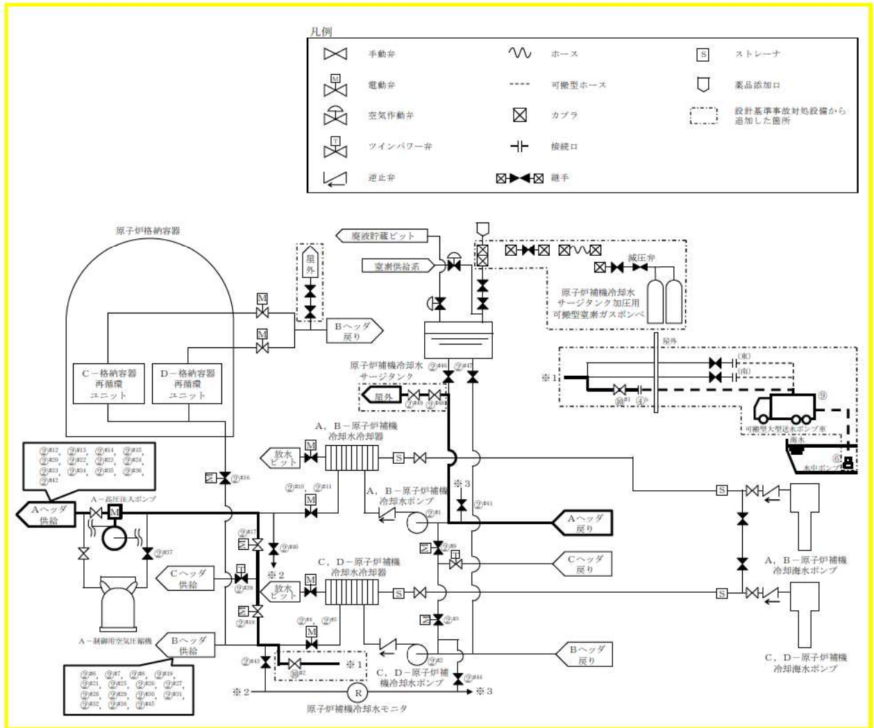
第 1.5.7 図 可搬型大型送水ポンプ車による A-高圧注入ポンプへの補機冷却水（海水）通水 概要図（3/4） （原子炉補助建屋西（建屋内）接続口を使用する場合（故意による大型航空機の衝突その他のテロリズムによる影響がある場合））
