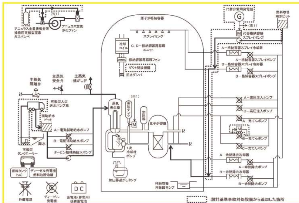
図4 「外部電源喪失時に非常用所内交流電源が喪失し、原子炉補機冷却機能の喪失する事故」の重大事故等対策の概略系統図 (2次冷却系強制冷却及び代替炉心注水)
