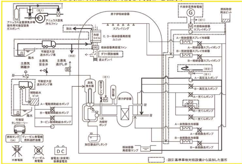
図2 「外部電源喪失時に非常用所内交流電源が喪失し、原子炉補機冷却機能の喪失及びRCPシールLOCAが発生する事故」の重大事故等対策の概略系統図 (格納容器内自然対流冷却及び高压代替再循環)
