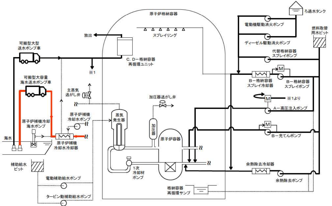
図2 概略系統図
