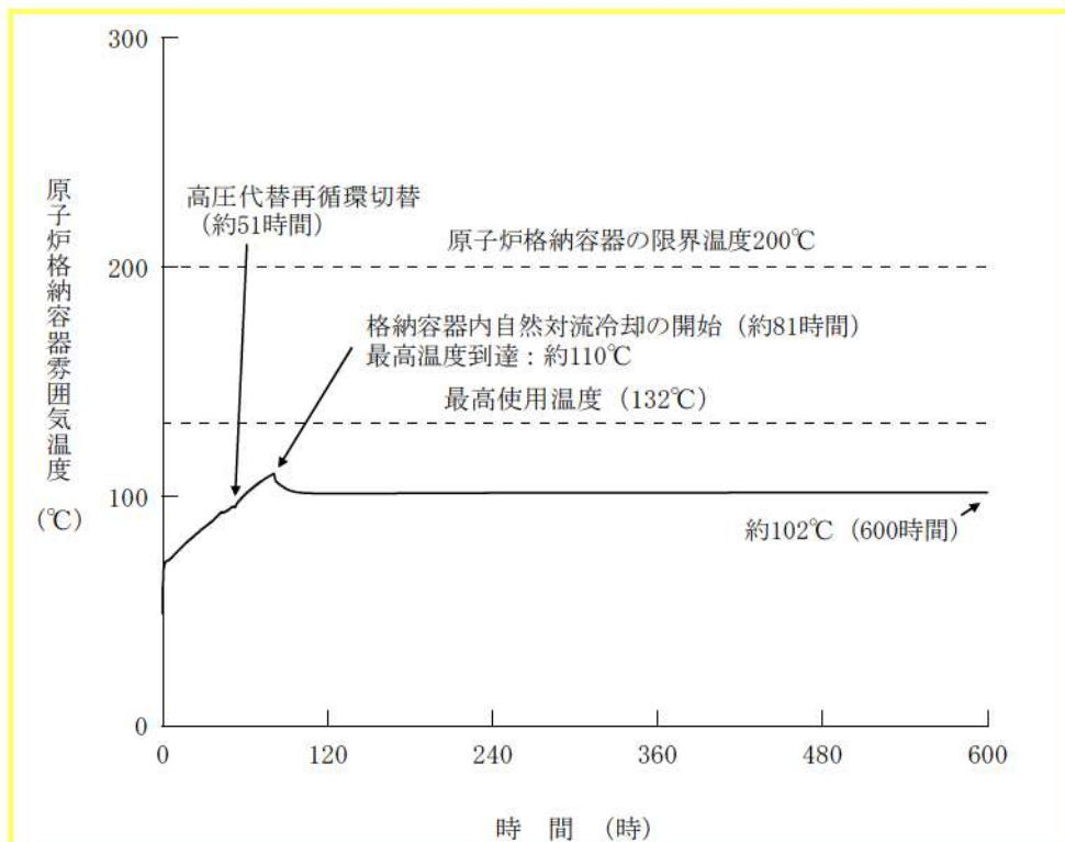
第 7. 1. 2. 27 図 原子炉格納容器雰囲気温度の長期間の推移 (RCP シール LOCA が発生する場合)
