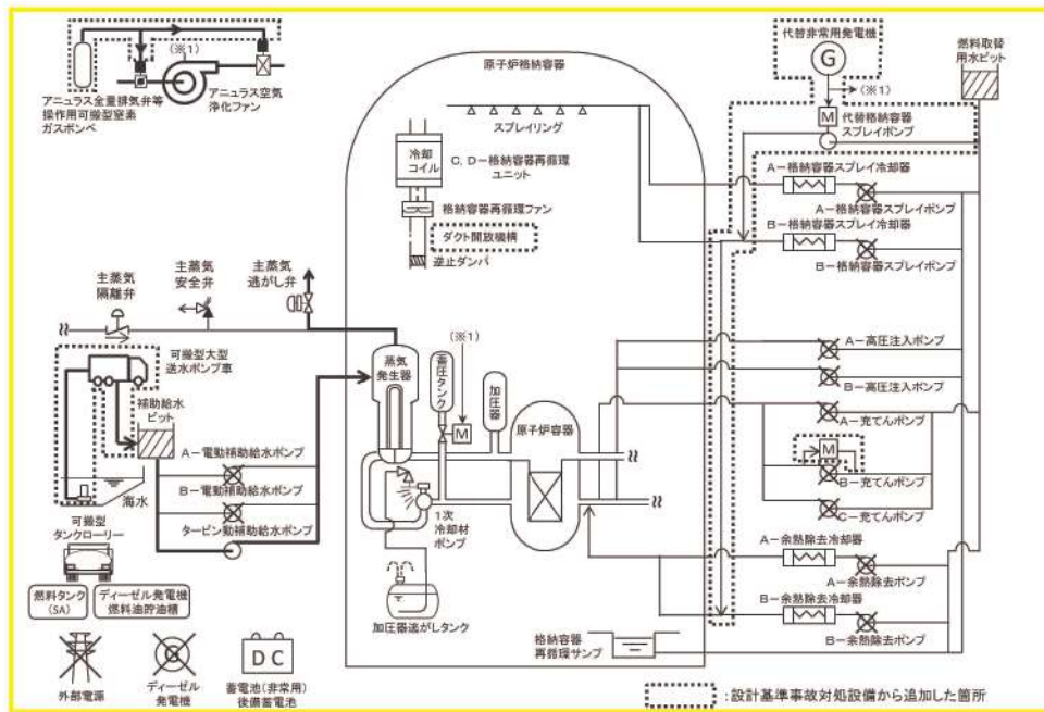
図3 「外部電源喪失時に非常用所内交流電源が喪失し、原子炉補機冷却機能の喪失する事故」の重大事故等対策の概略系統図 (2次冷却系強制冷却)
