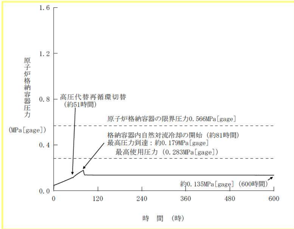
第 7. 1. 2. 26 図 原子炉格納容器圧力の長期間の推移 (RCP シール LOCA が発生する場合)
