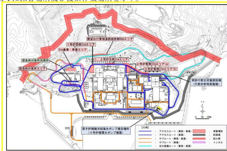
図4 保管場所及び復旧作業場所
