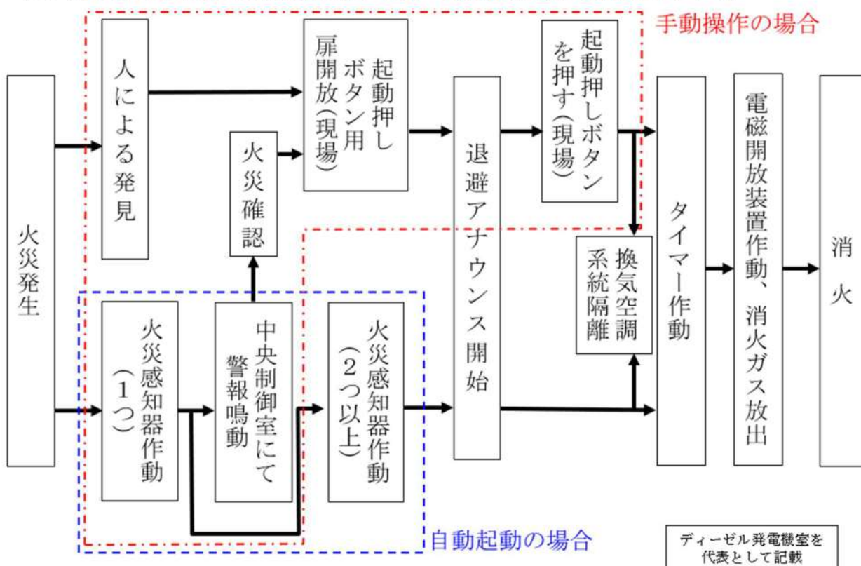
第2図：火災発生時の信号の流れ
