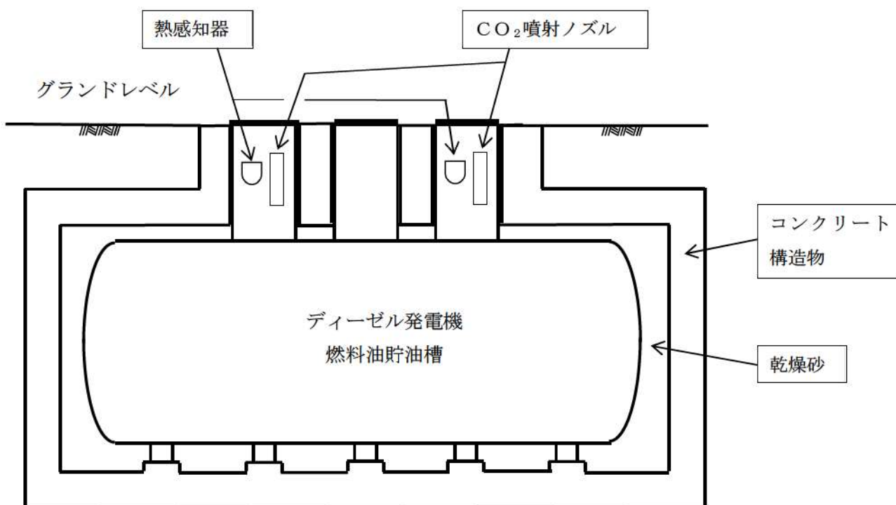
図1 ディーゼル発電機燃料油貯油槽概要図
