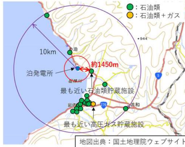
第 2. 2. 2. 2-1 図 泊発電所から 10km 圏内に位置する危険物施設
