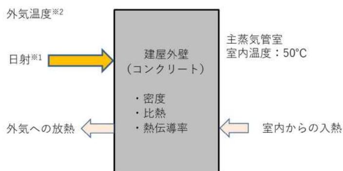
図 1 建屋外壁表面温度評価モデル
