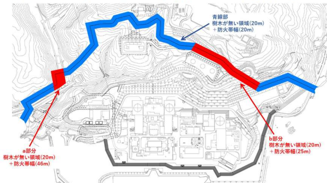
図1 防火帯位置
