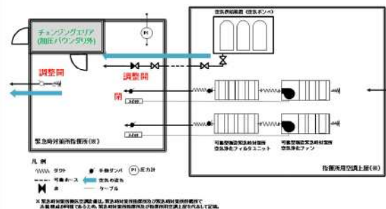
第1.18.22図 緊急時対策所換気空調設備 系統概要図 (ブルーム通過中：空気供給装置（空気ポンプ）による正圧化)
