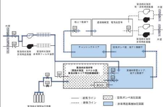
第2図 緊急時対策所換気空調系 系統概略図 (ブルーム通過中：緊急時対策所加压設備（空気ポンプ）による正圧化)
