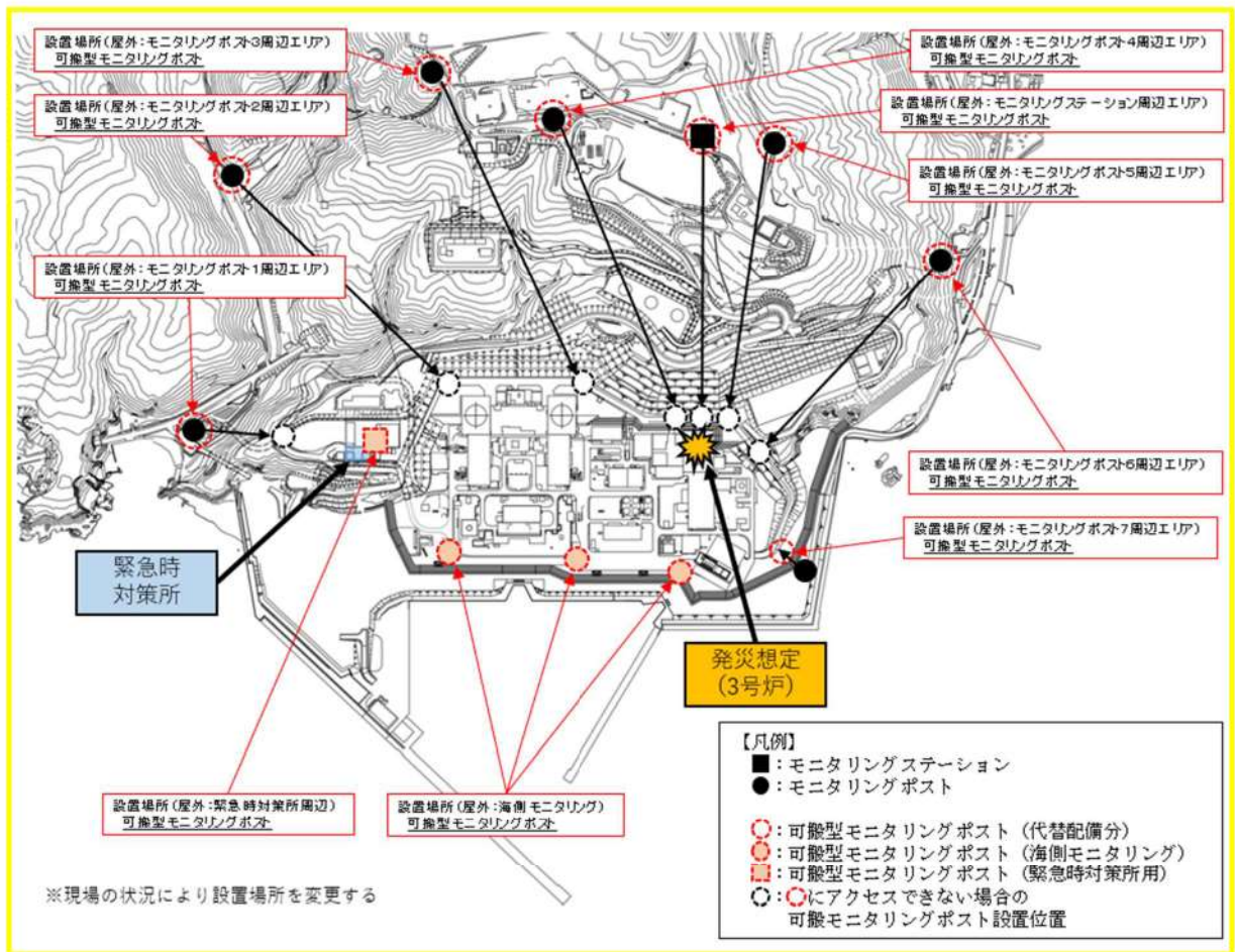
図添 14-2 プルームの状況を検知する手段
