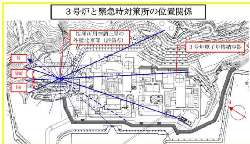
図添14-7 3号炉と緊急時対策所指揮所の位置関係
