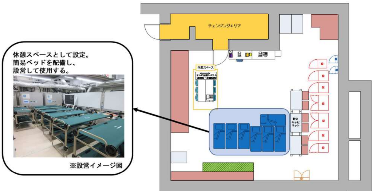
図 2.1-5 緊急時対策所待機所(休憩エリア) レイアウトイメージ図
