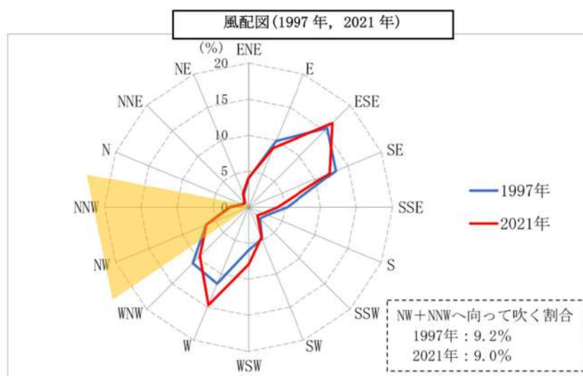
図2.4-21 風配図
