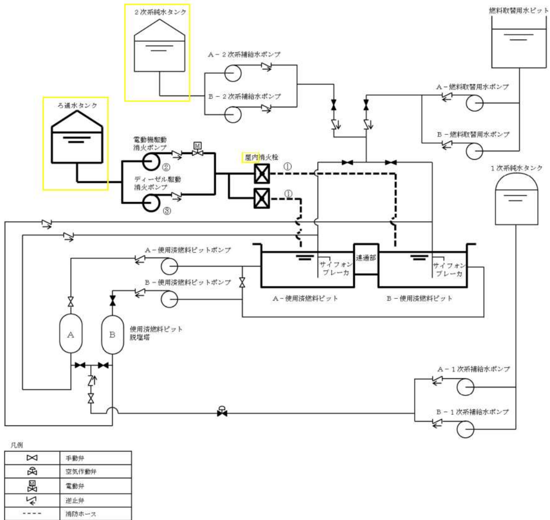
図 54-16-4 電動機駆動消火ポンプ又はディーゼル駆動消火ポンプによる使用済燃料ビットへの注水の概要図
