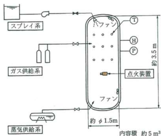
図4 試験装置
