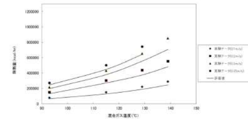
図5. 2-2 実験による検証試験データと除熱評価との比較 (図3. 2-1の横軸を変更したもの)
