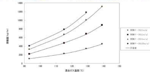
図5. 2-1 実験による検証試験データと凝縮量評価との比較 (図3. 2-2の横軸を変更したもの)
