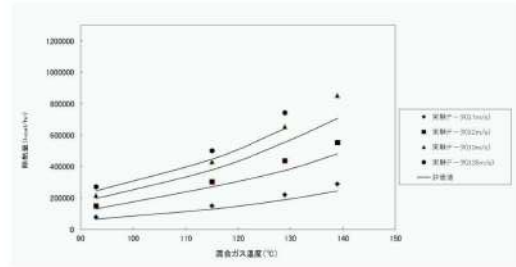
図5. 2-2 実験による検証試験データと除熱評価との比較 (図3. 2-1の横軸を変更したもの)
