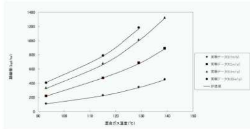
図5. 2-1 実験による検証試験データと凝縮量評価との比較 (図3. 2-2の横軸を変更したもの)
