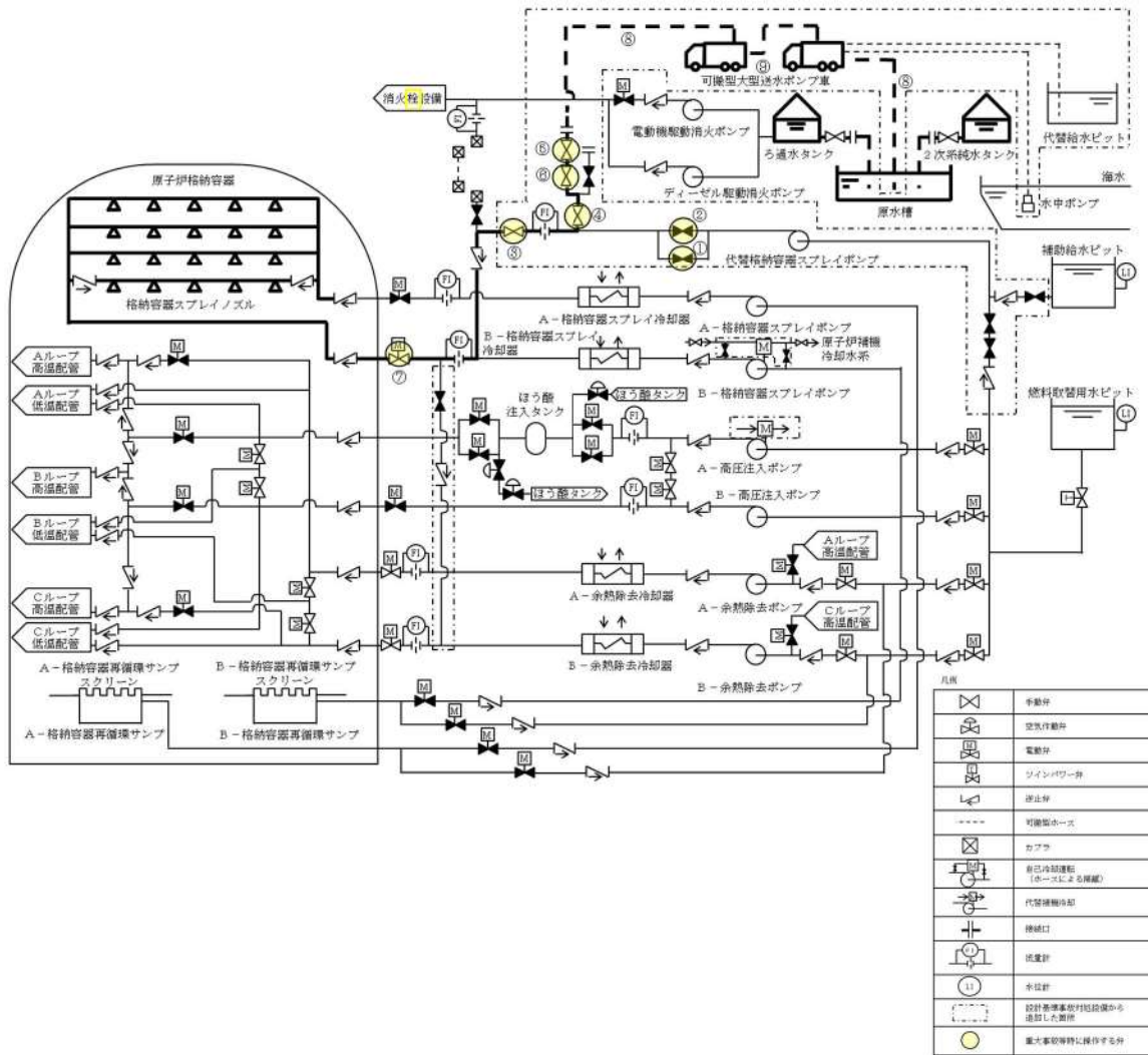
図 50-14-4 原水タンクを水源とした可搬型大型送水ポンプ車による原子炉格納容器内へのスプレイの概要図
