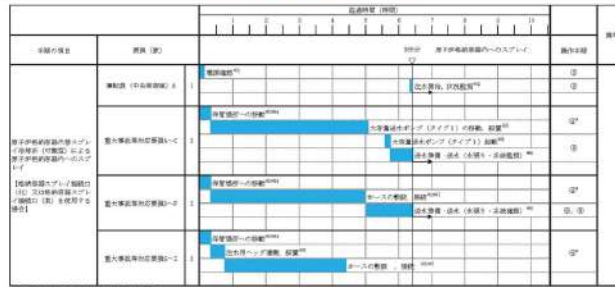
第1.6-14図 原子炉格納容器代替スプレイ冷却系（可搬型）による原子炉格納容器内へのスプレイ タイムチャート
