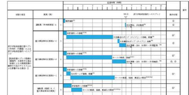
第1.6-16図 原子炉格納容器代替スプレイ冷却系（可搬型）による原子炉格納容器内へのスプレイ タイムチャート
