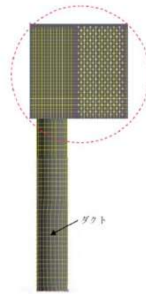
クーラー (ダクト有リ) メッシュ配置
