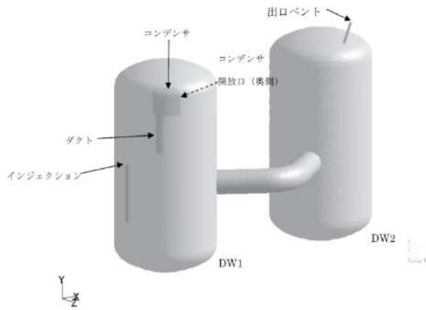
ST4-1 試験解析モデル (ダクト有リ上段配置)
