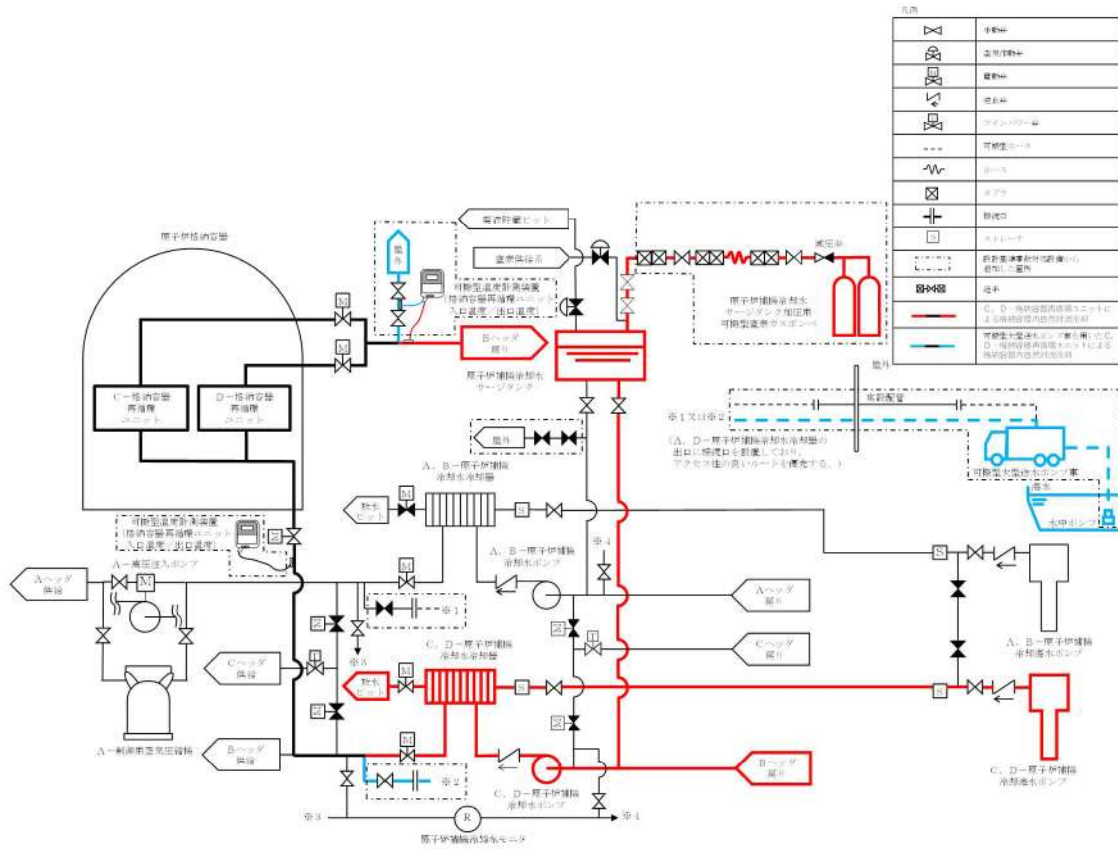
図1 格納容器内自然対流冷却システム概要図
