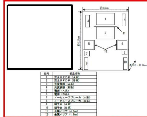
第7-3図 中央制御盤（安全系コンソール）内の構成部品配置
