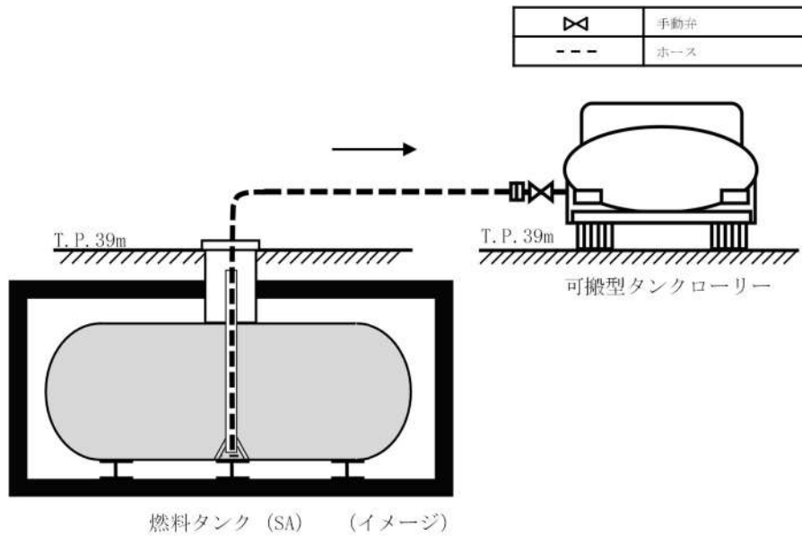
※：燃料タンク（SA）については、今後の検討により変更となる可能性がある。 第6図 燃料タンク（SA）から可搬型タンクローリー給油イメージ （可搬型タンクローリーによる直接汲み上げを行う場合）
