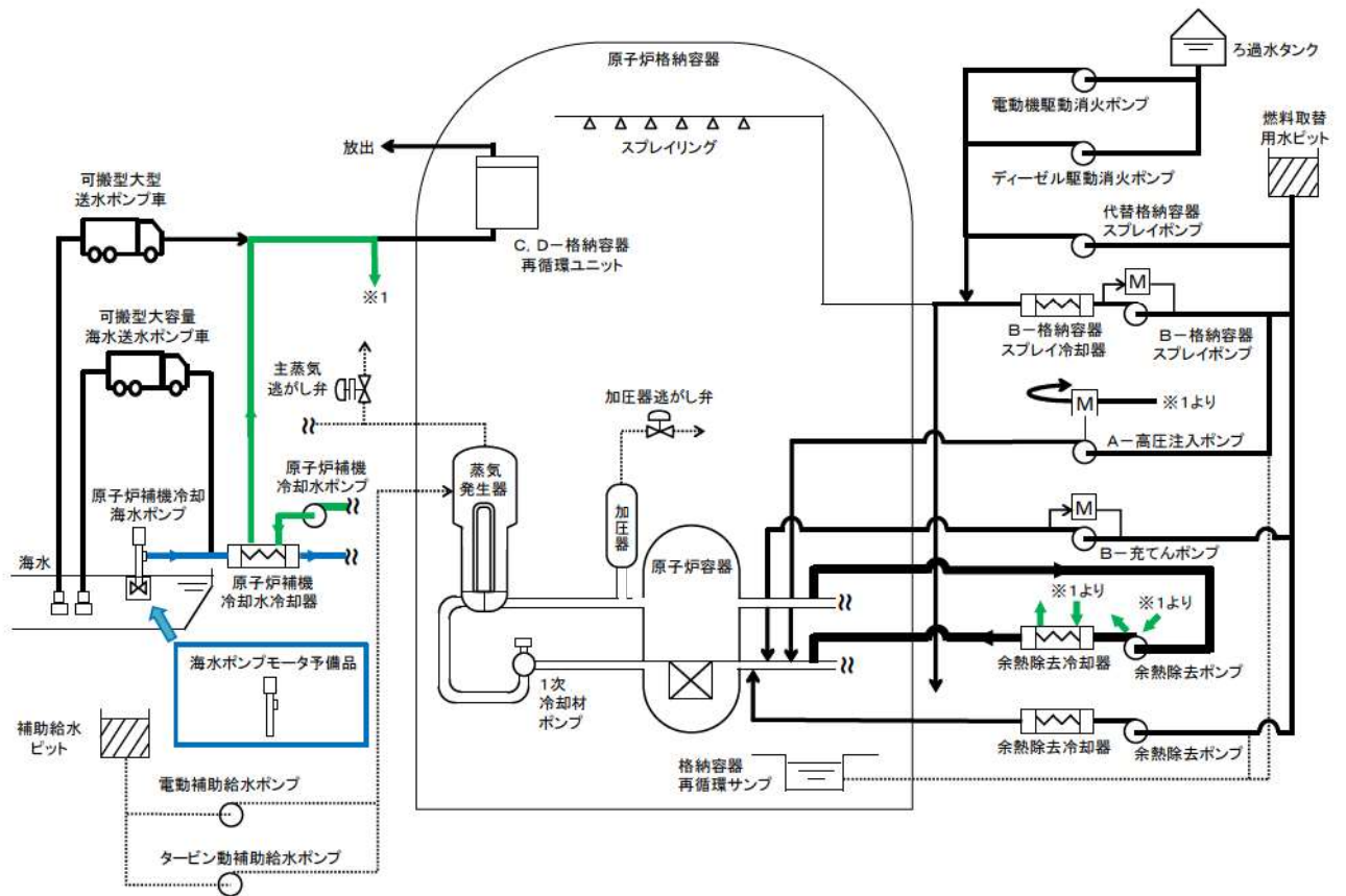
図5 概略系統図
