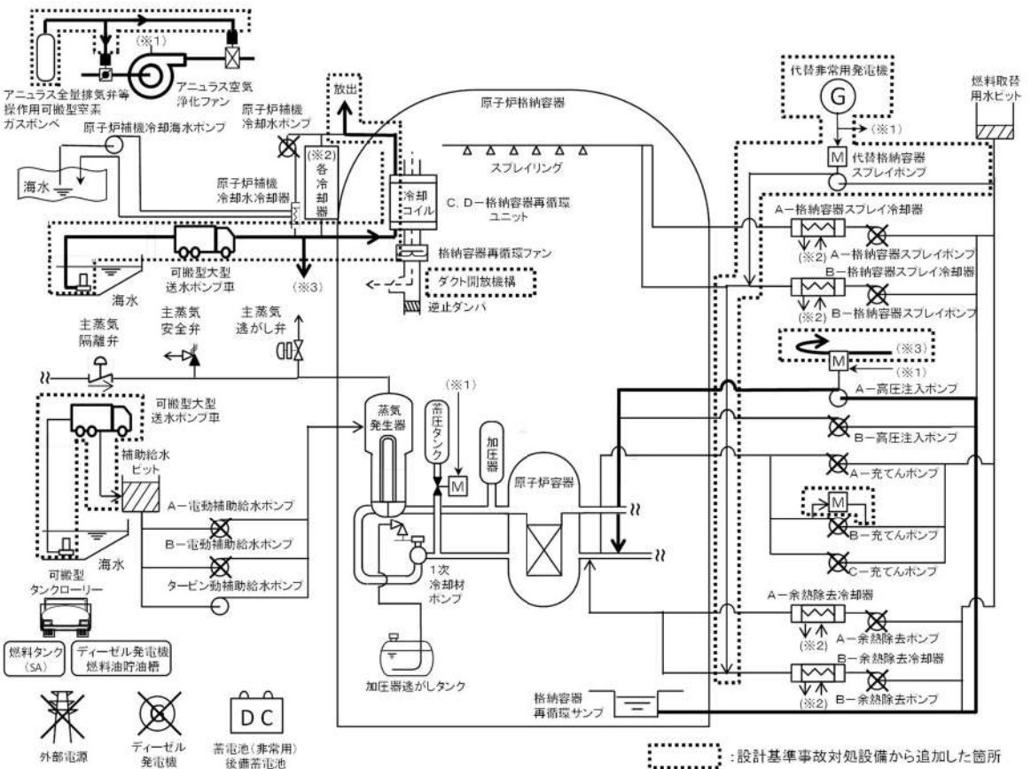
第 7.1.3.1 図 「原子炉補機冷却機能喪失」の重大事故等対策の概略系統図 (2/2) (高圧代替再循環及び格納容器内自然対流冷却)
