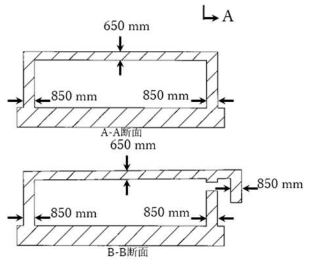
緊急時対策所待機所遮へい
