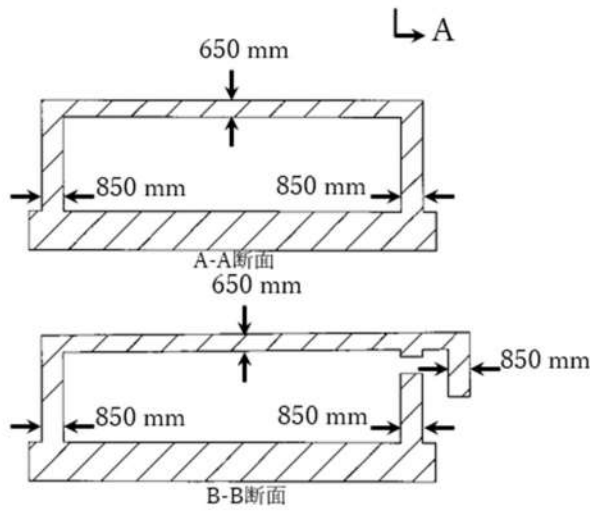
緊急時対策所指揮所遮へい
