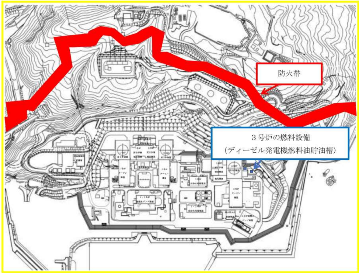
第 41-1-11 図：防火帯と燃料設備（ディーゼル発電機燃料油貯油槽）の位置関係
