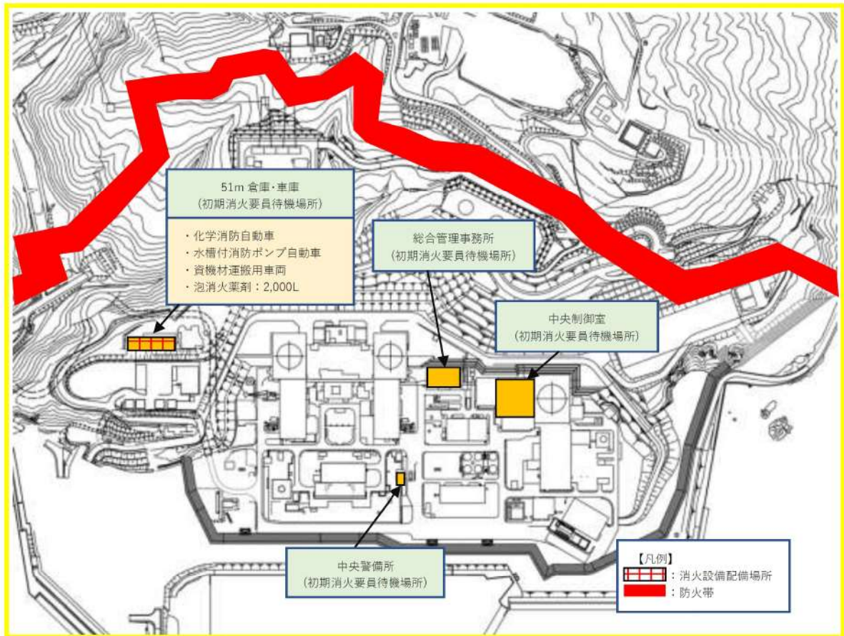
第 41-1-16 図：移動式消火設備の配置の概要
