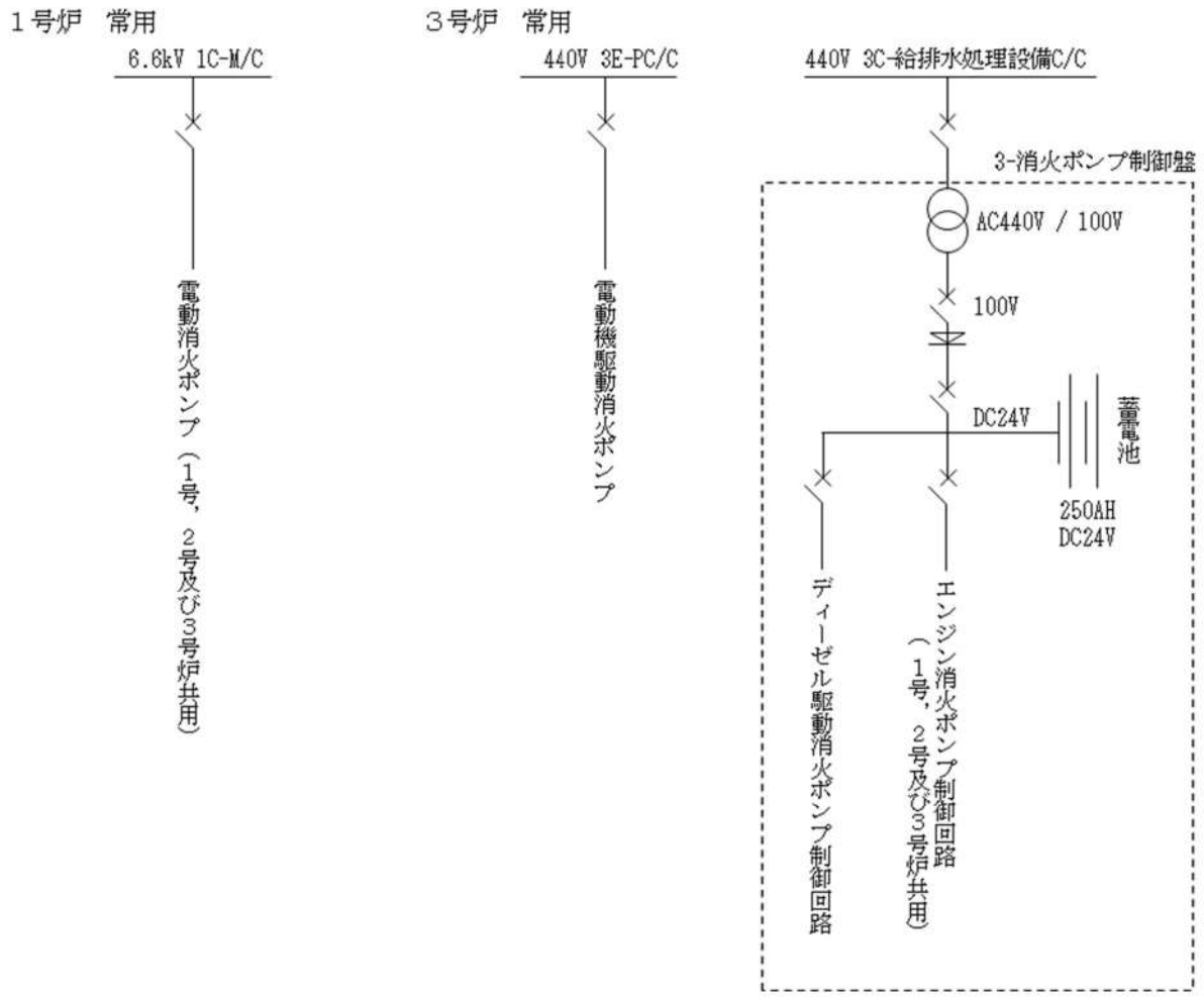
第 41-1-17 図 : 消火設備電源の概要
