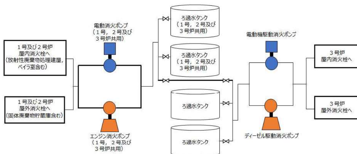
第41-1-14図：消火用水供給系の概要
