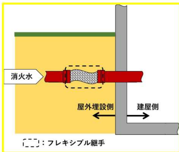
第 41-1-23 図 地盤変位対策の実施例
