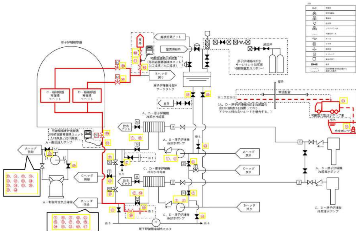
図 49-4-3 格納容器内自然対流冷却
