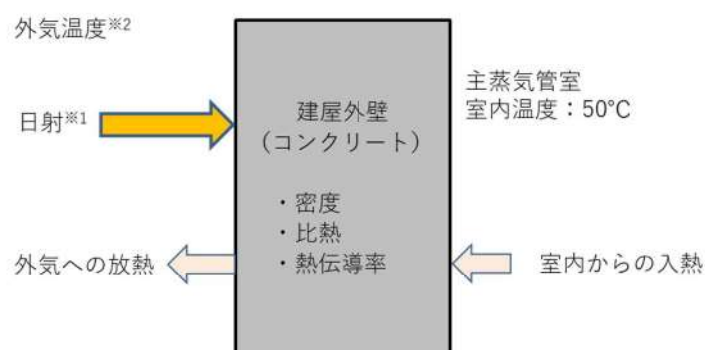
図 1 建屋外壁表面温度評価モデル
