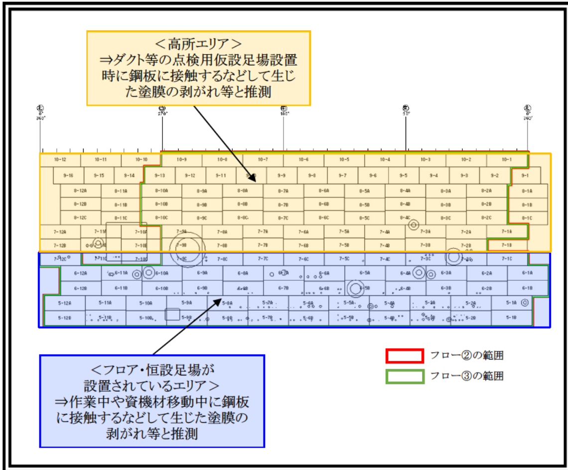
図 5. 3 軽微な劣化が確認された範囲（円筒部外面）
