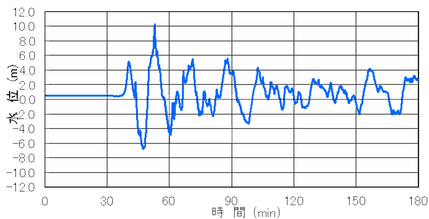
第 3.1.4.2.2.12 図 遡上解析で想定する入力津波の時刻歴波形 (鋸崎から約 1km 離れた海域 (水深 40m 地点)) (3, 4号機海水ポンプ室前潮位 : E.L. + 15.8m) (初期潮位 : E.L. + 0.49m)
