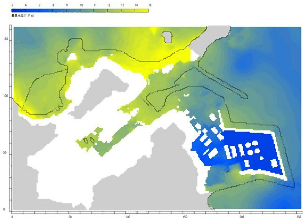
第 3.1.4.2.2.3 図 最高水位分布 ( 3 , 4 号機海水ポンプ室前潮位 : E.L. + 11.4m )
