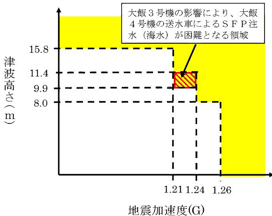
第 3.1.4.4.1.4 図 大飯 3 号機からの影響を考慮した大飯 4 号機の地震と津波の重畳に関するクリフエッジ評価結果（SFP燃料損傷）
