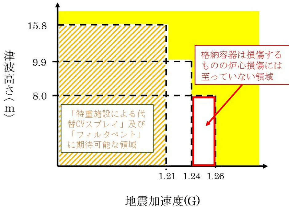
第 3.1.4.2.3.8 図 遡上を考慮した地震と津波の重畳に関するクリフエッジ評価結果（格納容器損傷）
