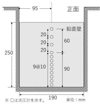
図1 水路及び堤体の概要
