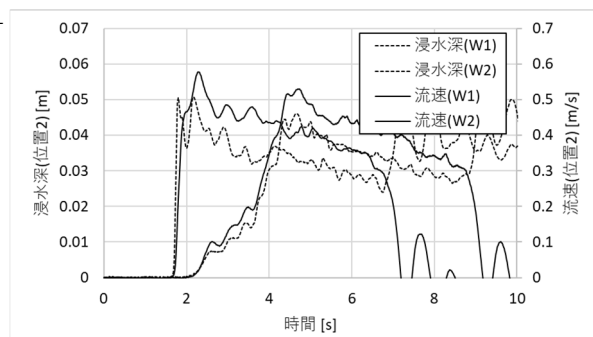
図2 波形の概要 (位置2)
