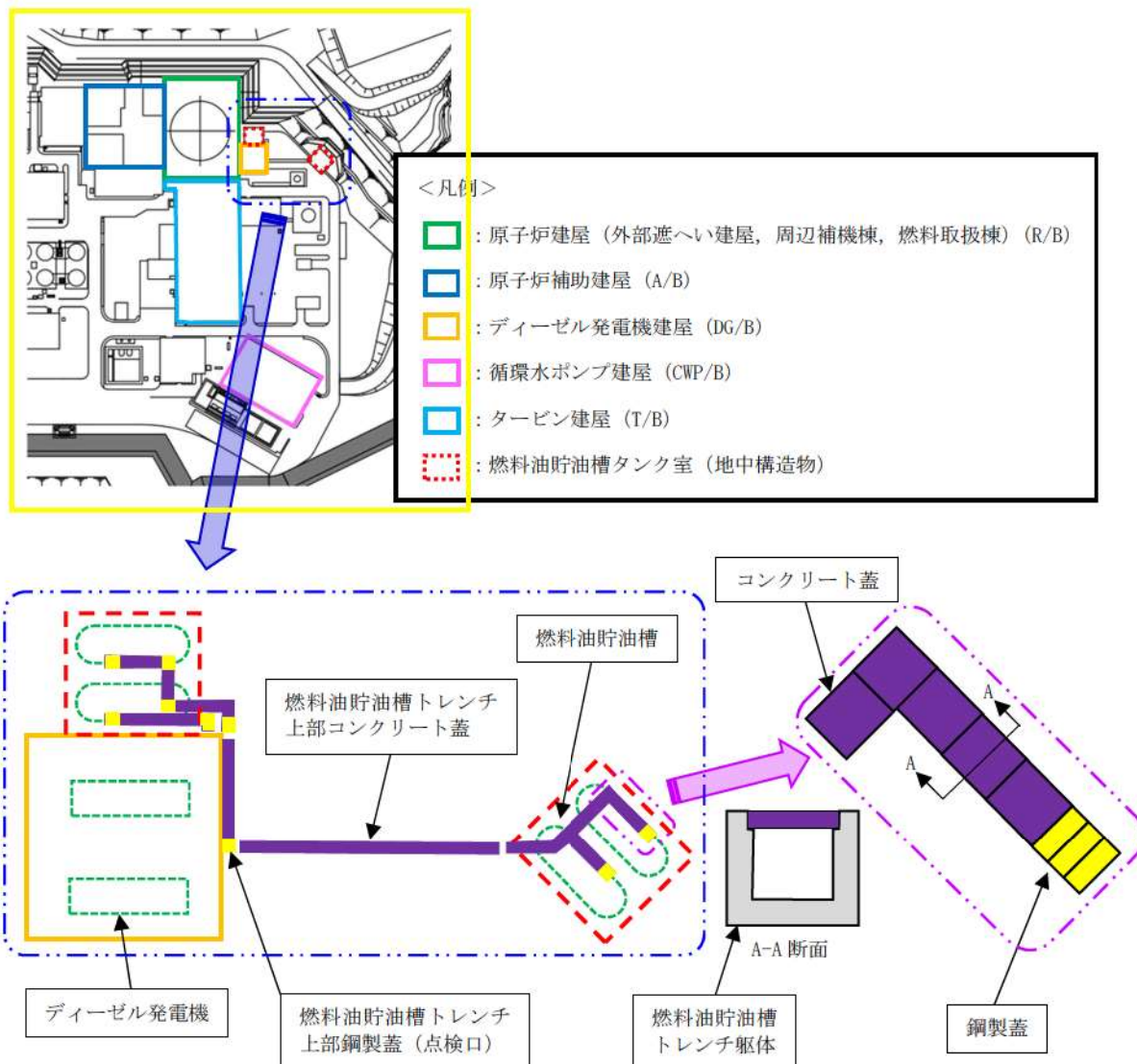
図1 燃料油貯油槽トレンチ上部のコンクリート蓋及び鋼製蓋の概略配置図
