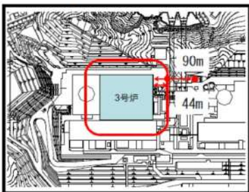
図2：航空機落下地点と補助ボイラ燃料タンク的位置関係
