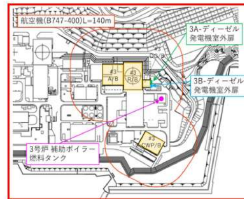
図6-15 想定する3号炉補助ボイラー燃料タンクと航空機墜落による火災の火災源と3B-ディーゼル発電機室外屏の位置図
