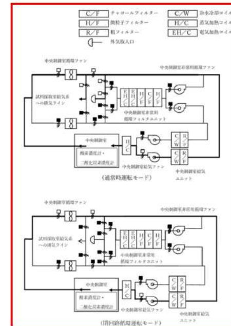
図8-2(d) 中央制御室換気空調装置系統概要図
