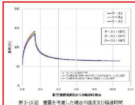
第2-19図 重量を考慮した場合の温度及び経過時間
