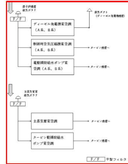
図8-2(c) 原子炉建屋換気空調設備全体概要図
