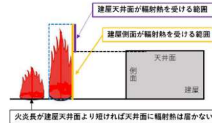
図5-4 建屋天井面の評価概念図
