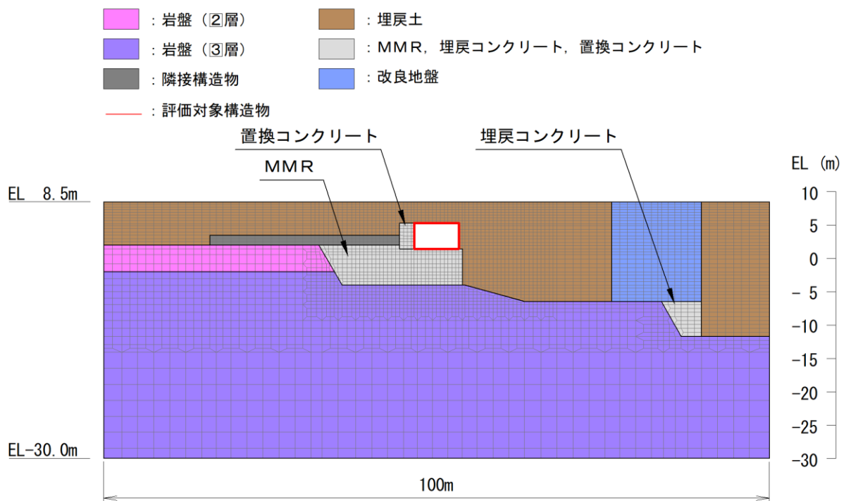
図 3-11(5) 屋外配管ダクト (タービン建物～放水槽) 地震応答解析モデル (E W断面 (C-C断面*))
