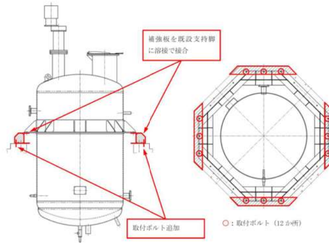
ほう酸補給タンクの工事内容
