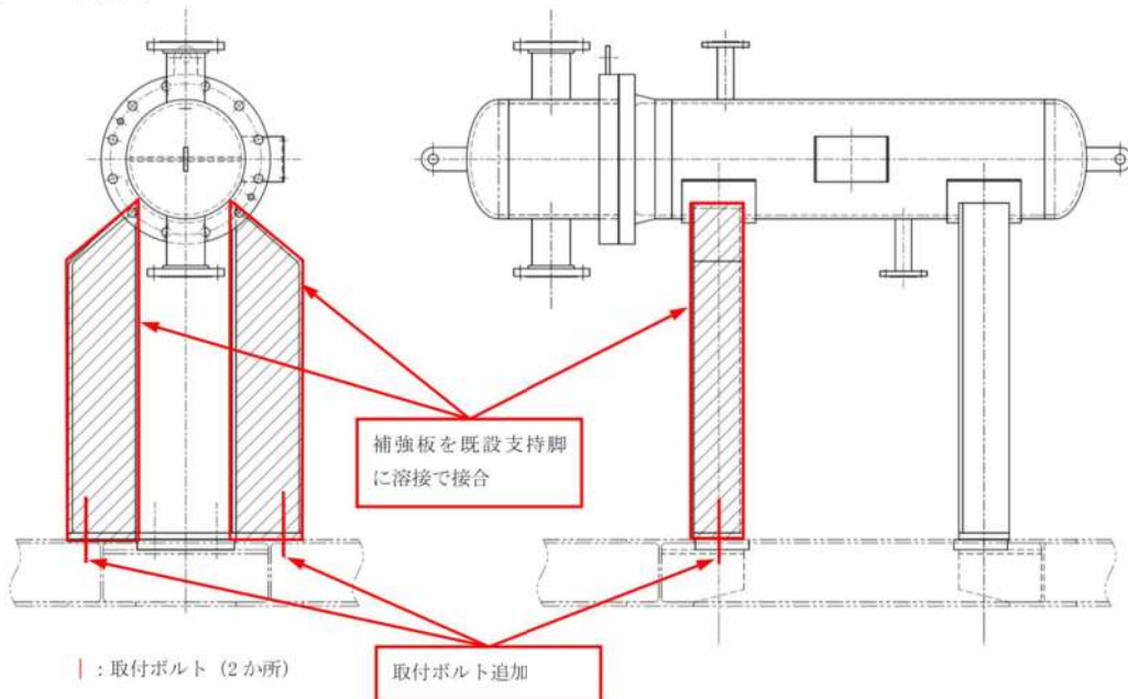
燃料取替用水加熱器の工事内容
