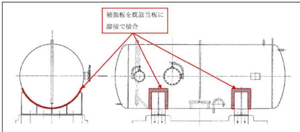
洗浄排水タンクの工事内容
